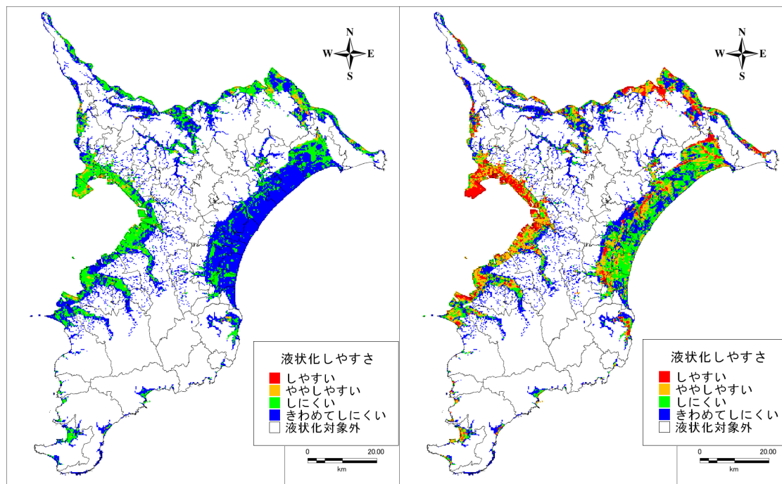
震度 5 弱
