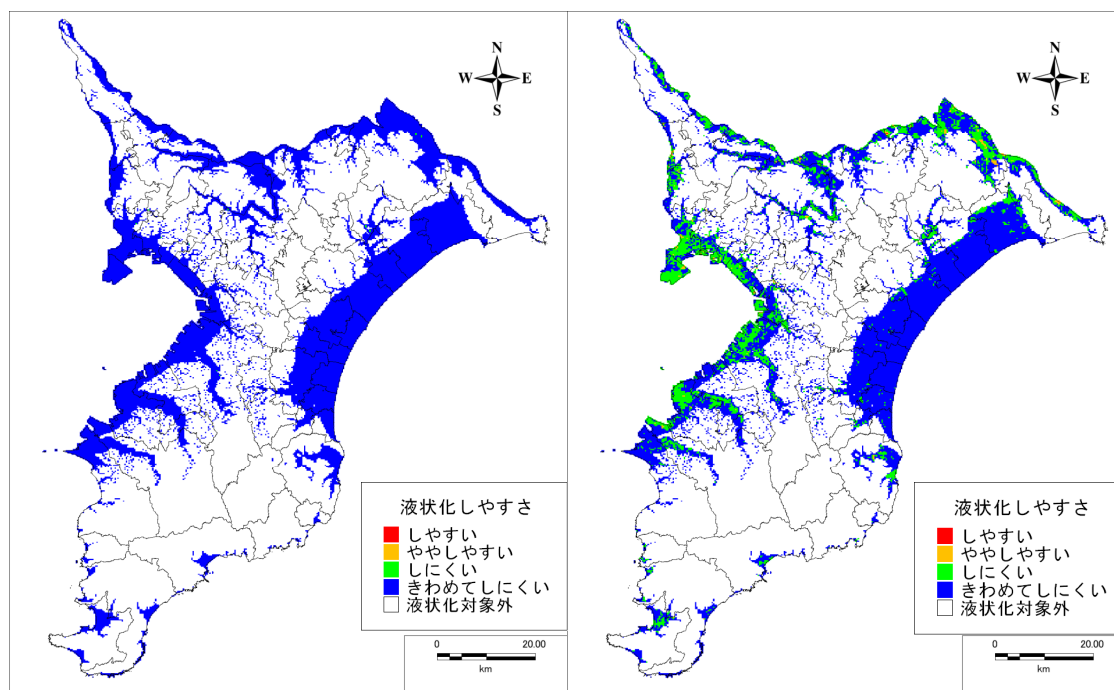
震度 5 弱
