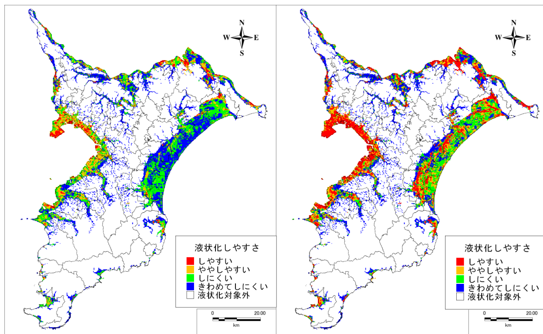
震度 6 弱
