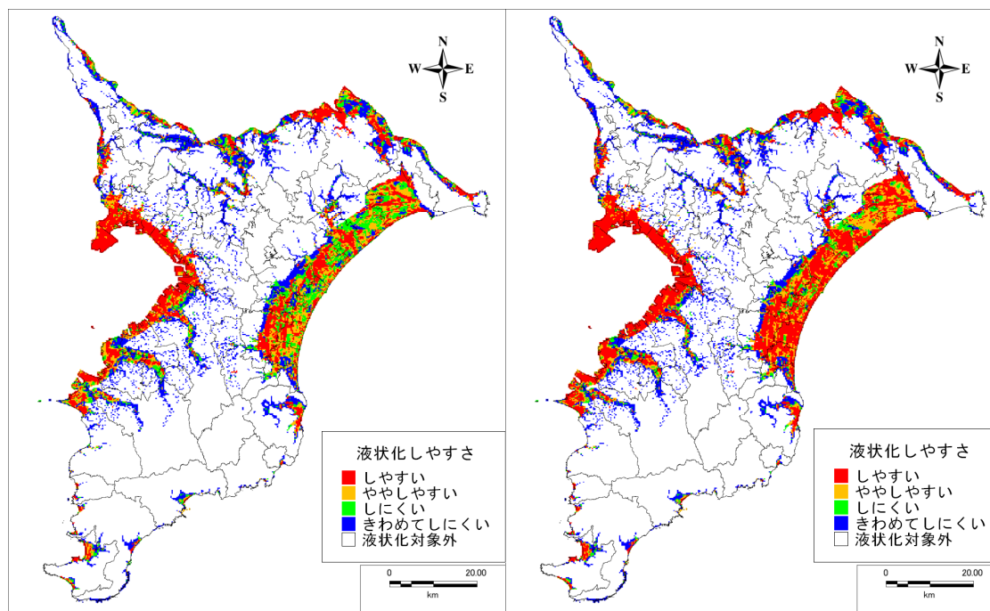
震度 6 弱
