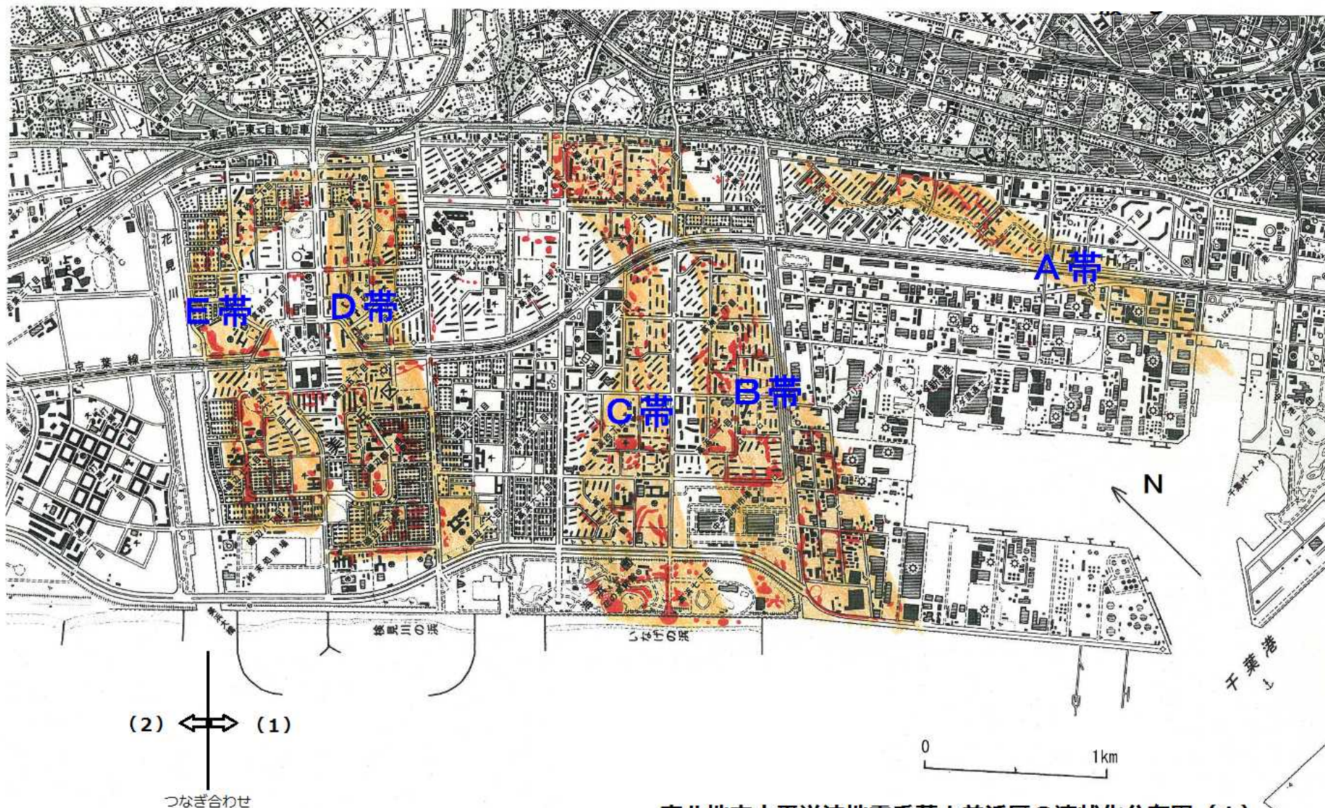
東北地方太平洋沖地震千葉市美浜区の液状化分布図 (1)
