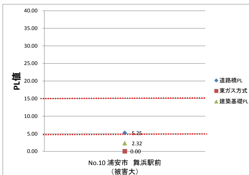
図 3.2-6 浦安市舞浜駅前のボーリング地点（南西ー北東）における道路橋，東京ガス方式，建築基 礎による PL 値
