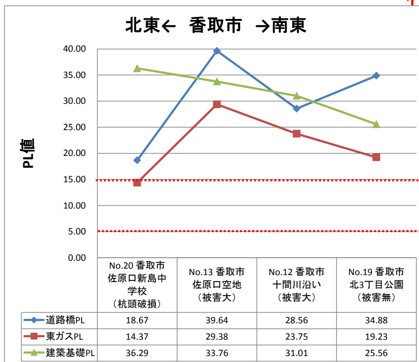
図 3.2-5 香取市のボーリング地点（南西ー北東）における道路橋，東京ガス方式， 建築基礎による PL 値
