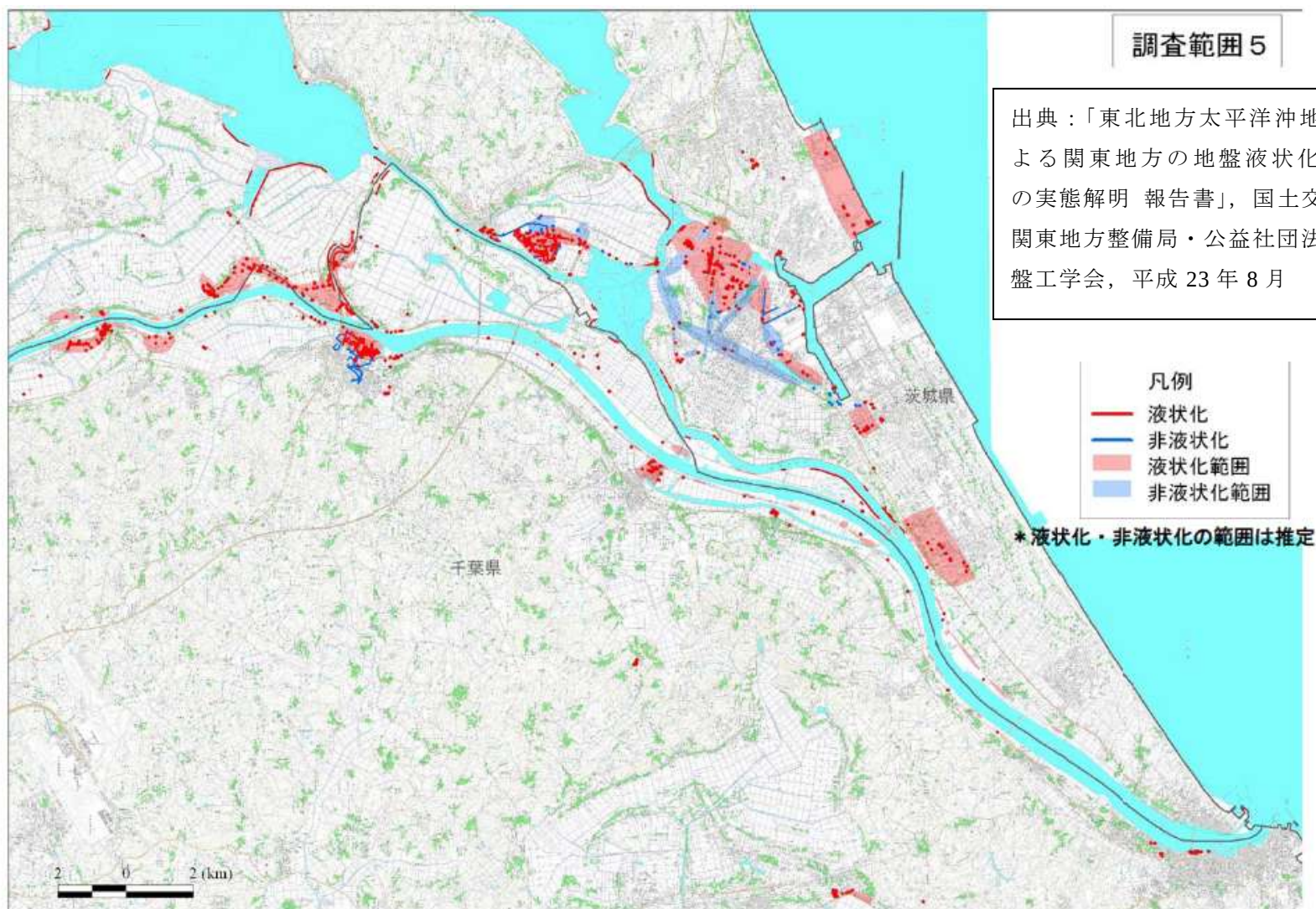
図 2.3-7 液状化調査範囲位置図その 5（利根川下流域（佐倉～銚子），霞ヶ浦南東部）
