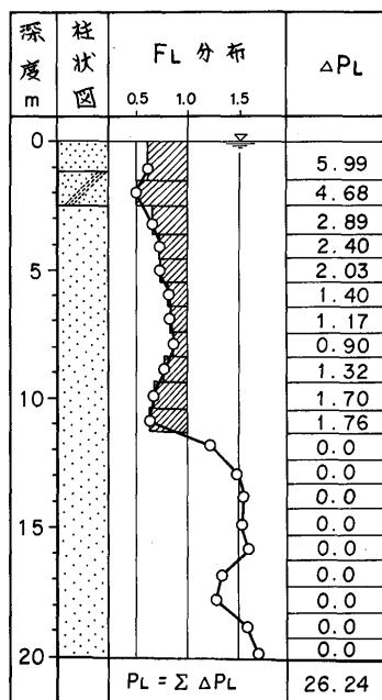
図 3.2-1 P_1 法の概要 (岩崎他(1980)に加筆)
