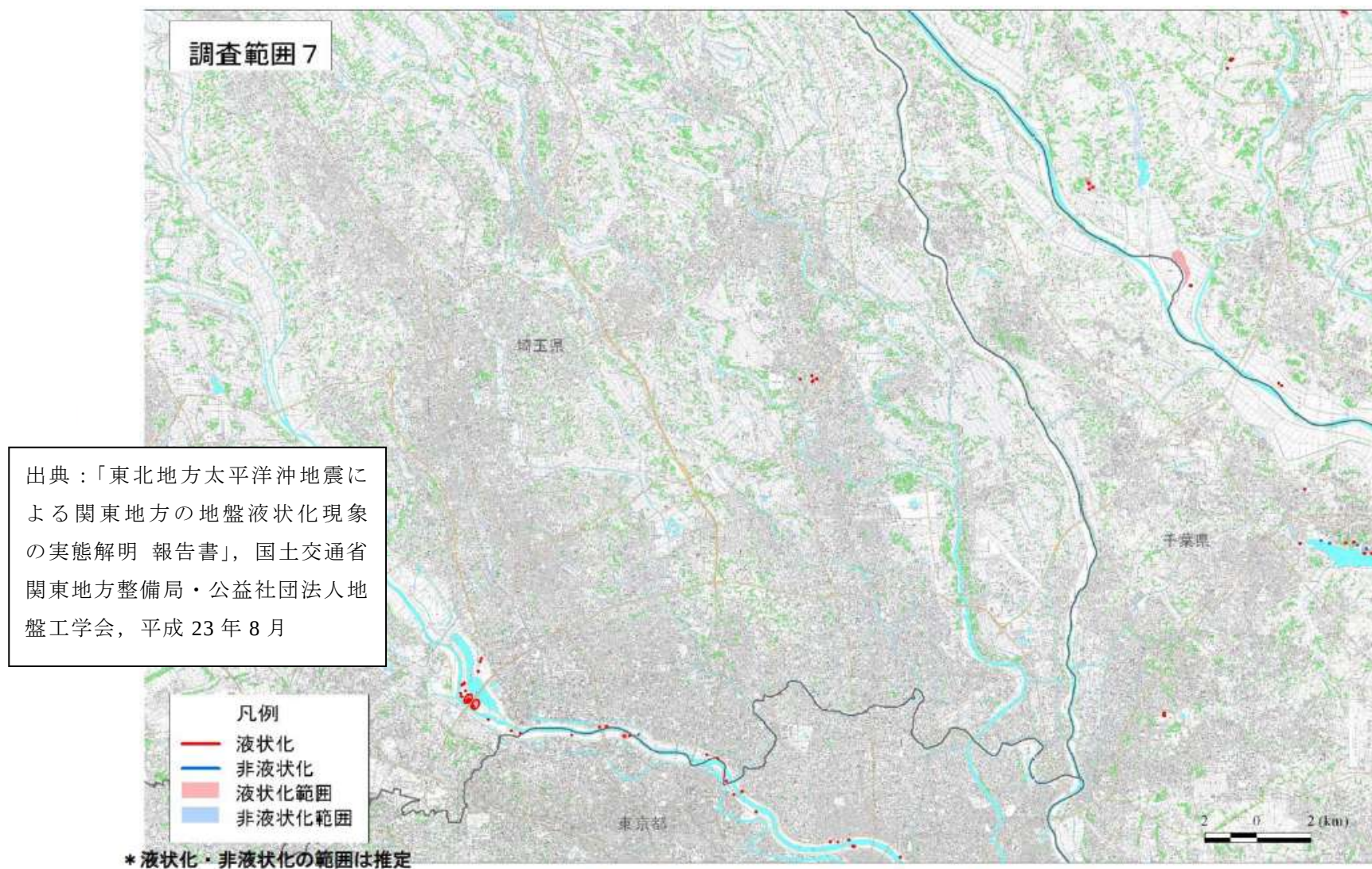
図 2.3-9 液状化調査範囲位置図その 7（荒川下流北部，古利根川流域南部）
