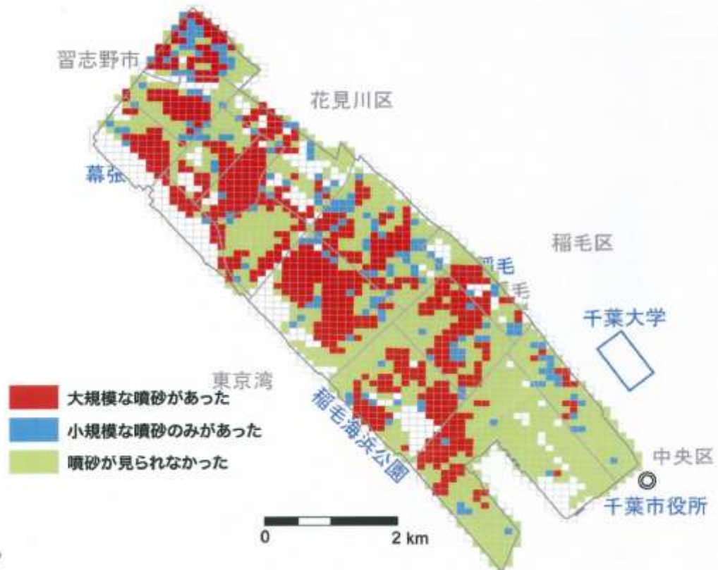
図 3. 2-2 (3) 千葉大学・中井教授らの調査による美浜区の液状化被害（噴砂）の分布
