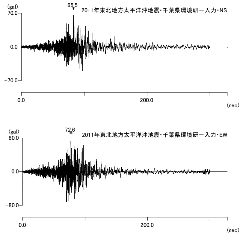
図 3.7-2 2011 年東北地方太平洋沖地震の工学的基盤面における入力波形
