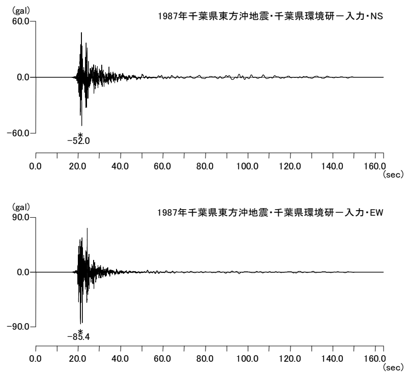
図 3.7-3 1987 年千葉県東方沖地震の工学的基盤面における入力波形
