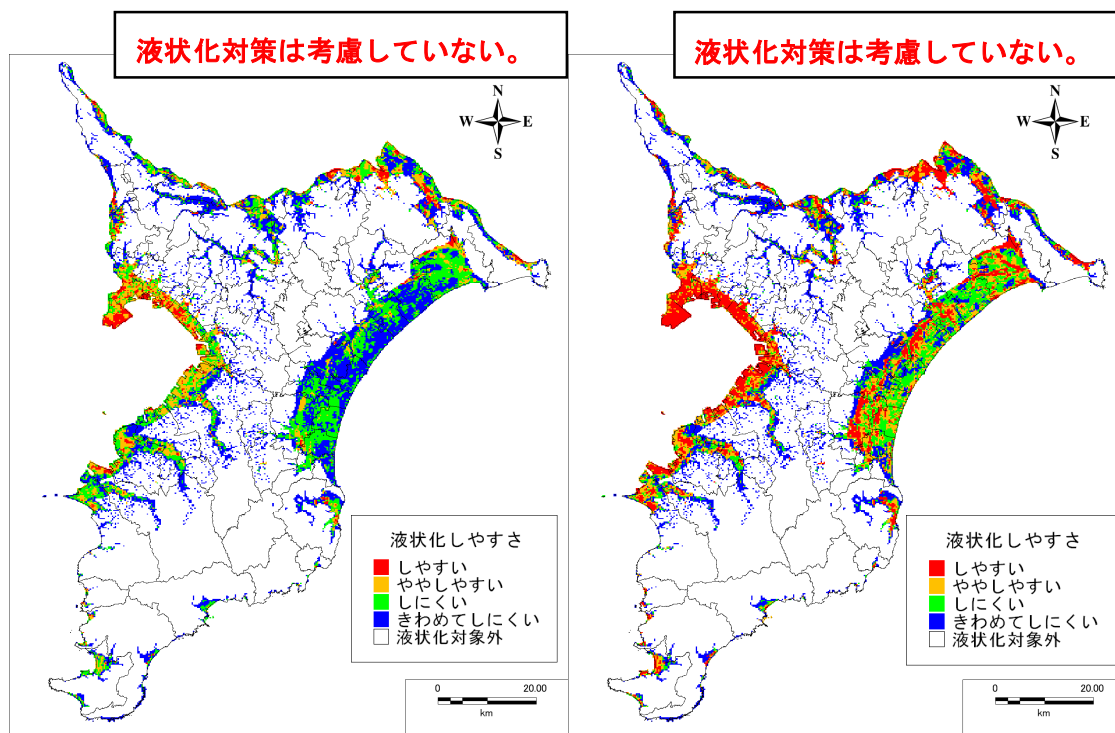
図 5-10 液状化しやすさ（直下地震）
