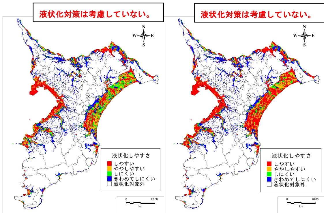
図 5-11 液状化しやすさ（超巨大地震）
