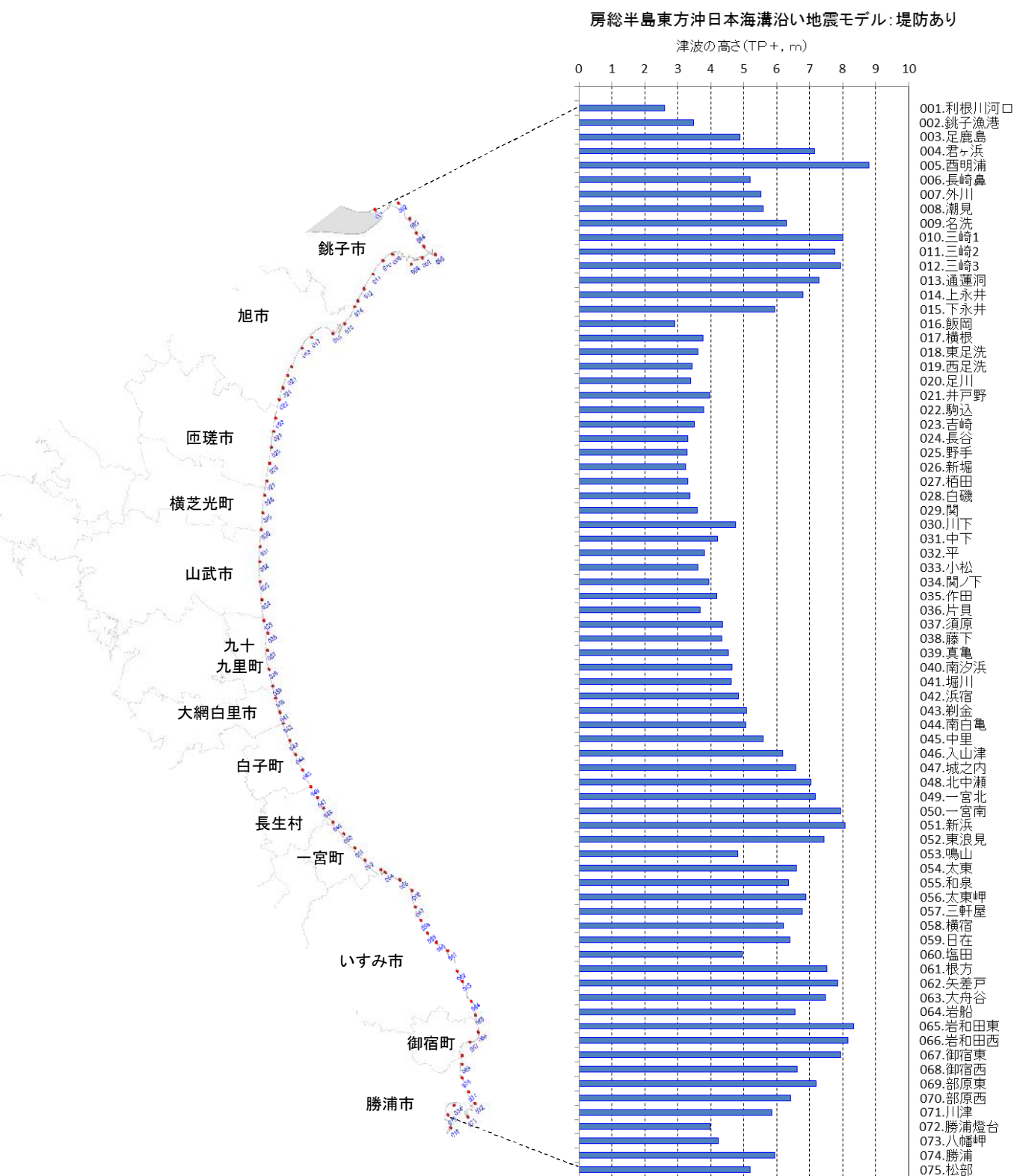
図 8-28 水位出力地点における最大津波高の比較 (堤防あり)
