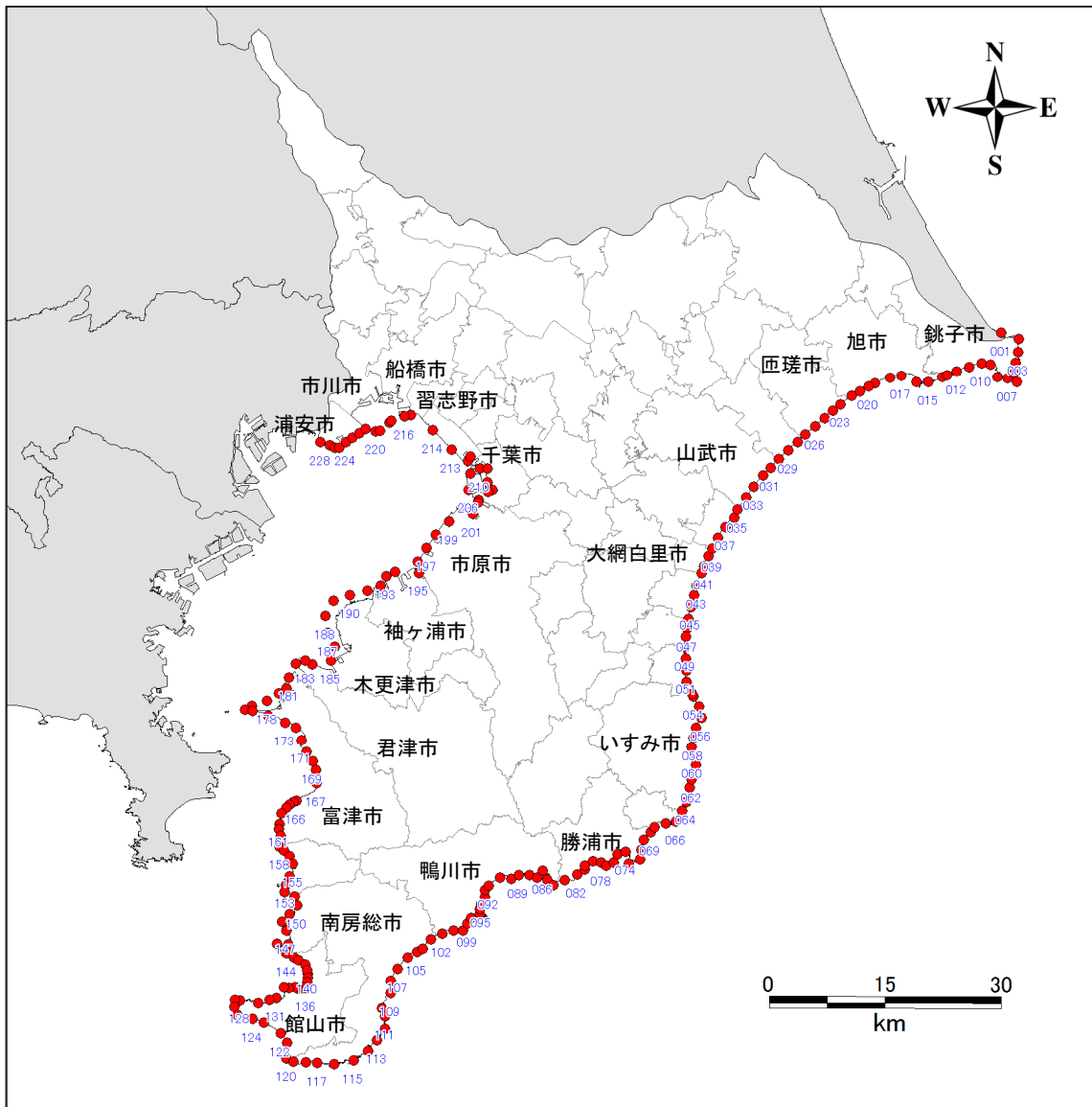
図 8-23 水位出力地点（228 点）
