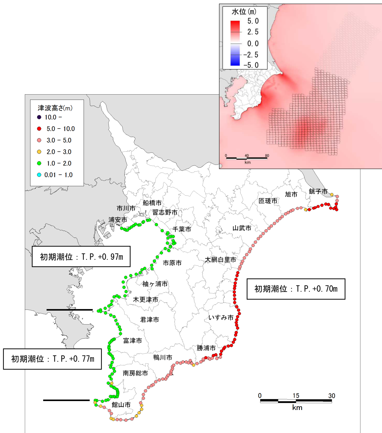
図 8-25 水位出力地点における最大津波高の分布(堤防あり)
