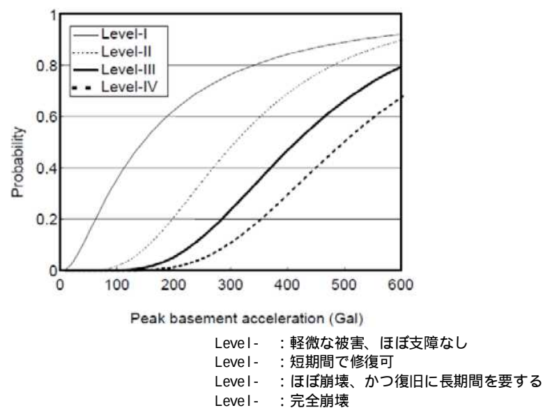
図13-6 港湾岸壁被害確率の累積分布関数（ICHI 2004 59 ）
