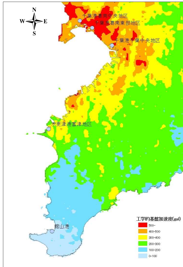
図13-7 港湾施設と地震動（工学的基盤加速度）との関係（千葉県北西部直下地震）
