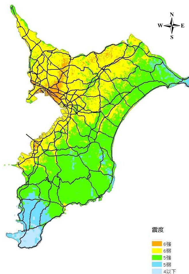
図13-2 緊急輸送道路と震度との関係（千葉県北西部直下地震）
