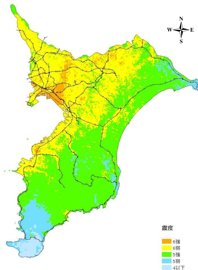
図13-4 鉄道施設と震度との関係（千葉県北西部直下地震）
