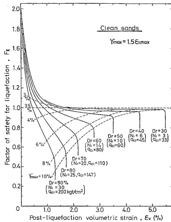
図14-10 Ishihara and Yoshimine(1992)による F_L 値と体積圧縮ひずみの関係
