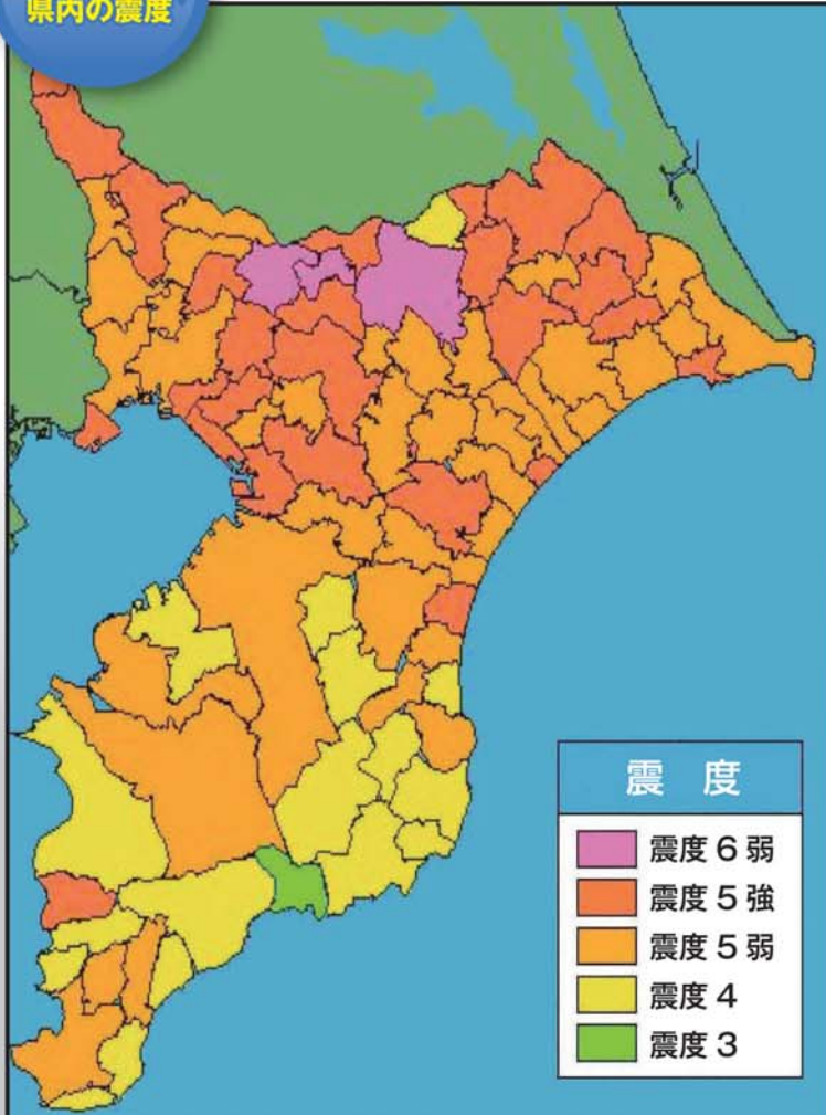
千葉県の市町村別震度分布図
