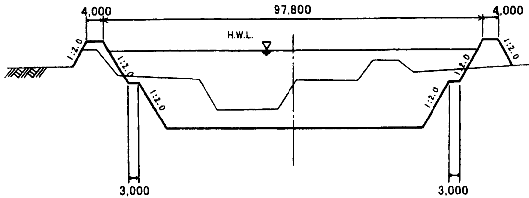
標準断面図
