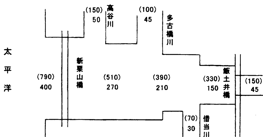
計画流量配分図
