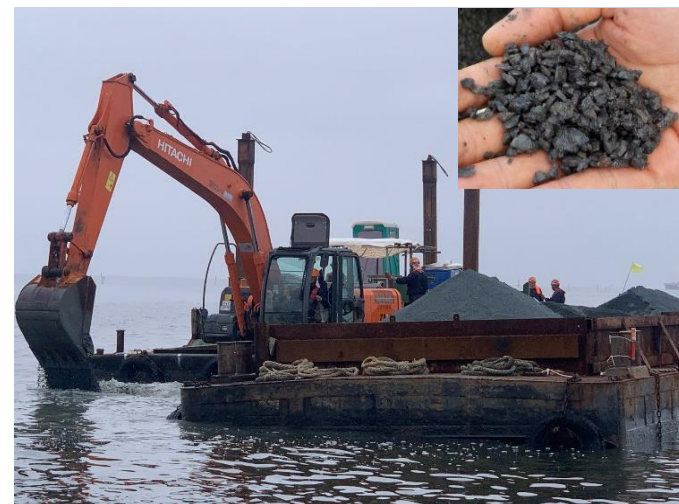
図 2 碎石覆砂実施状況 (船橋市漁業協同組合活動グループ)
