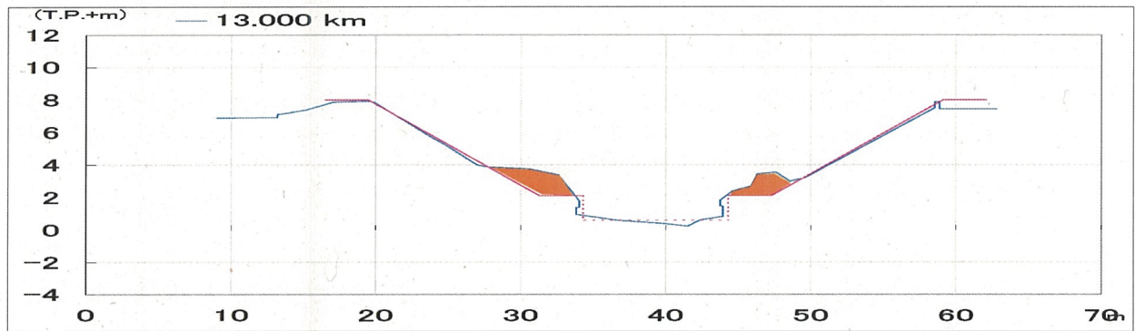
横断面と堆積土砂イメージ
