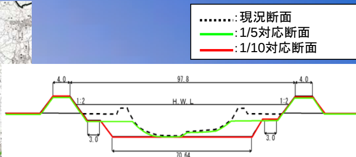
栗山川標準横断面図
