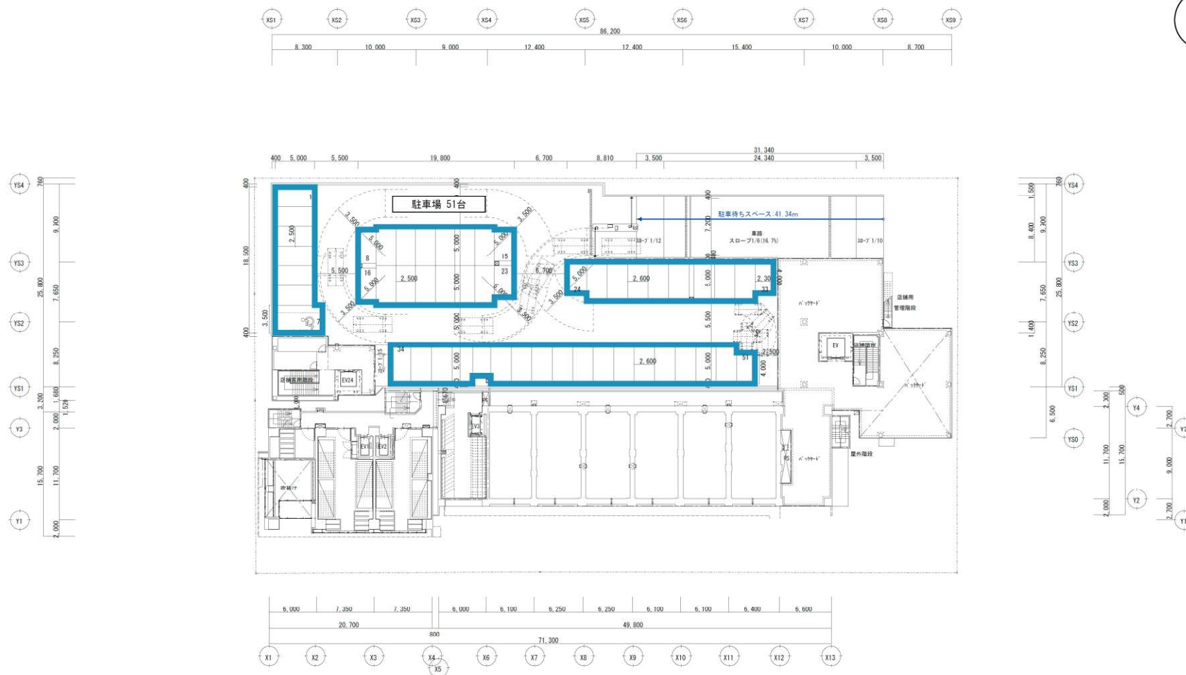
図4 2階平面図
