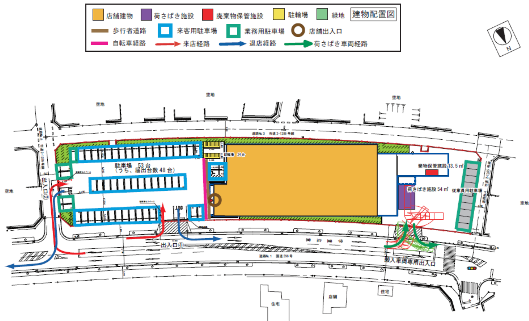
図3 建物配置図
