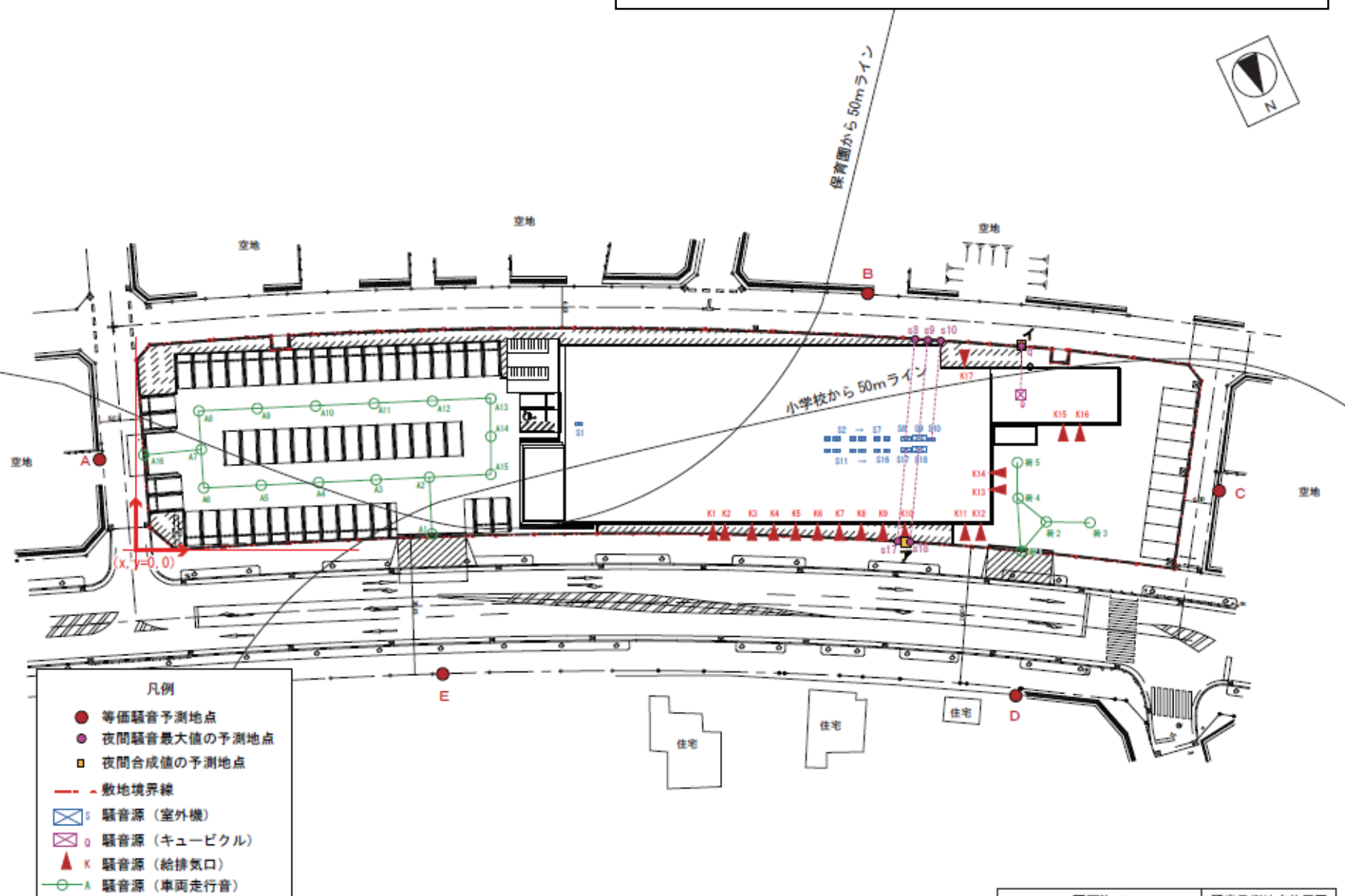
図5 騒音発生予測地点位置図
