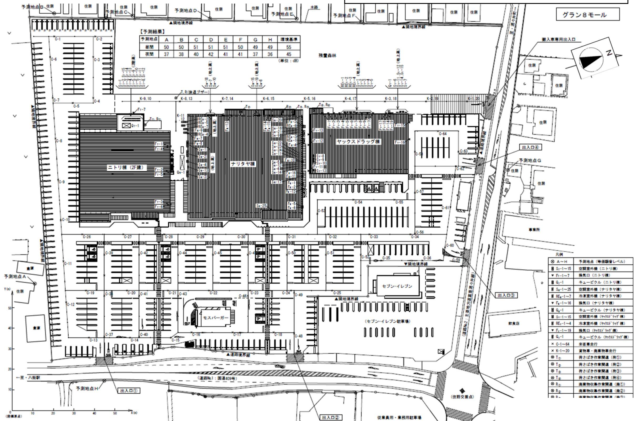
図5 騒音発生源及び予測地点位置図
