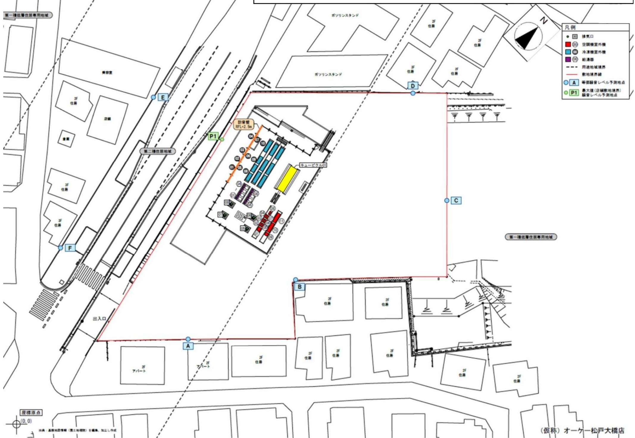
図5-4 騒音発生源及び予測地点位置図(PH階)
