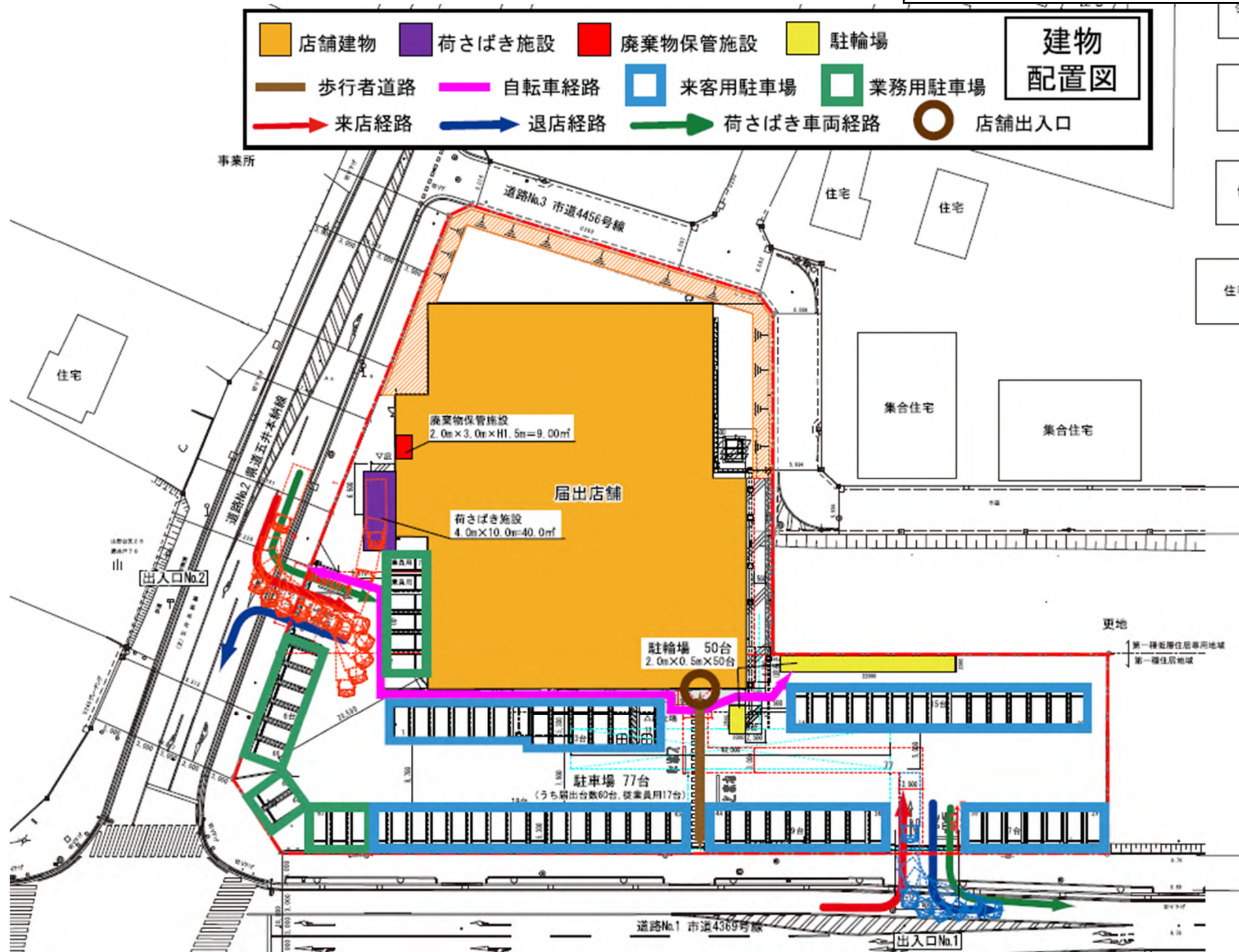
図3 建物配置図
