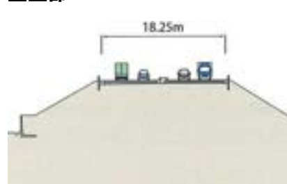
盛土部
