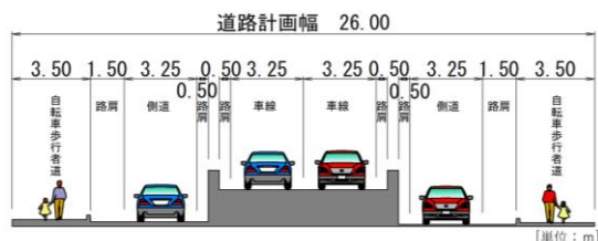
【取付部断面】
