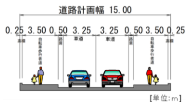
【渡河部断面】
