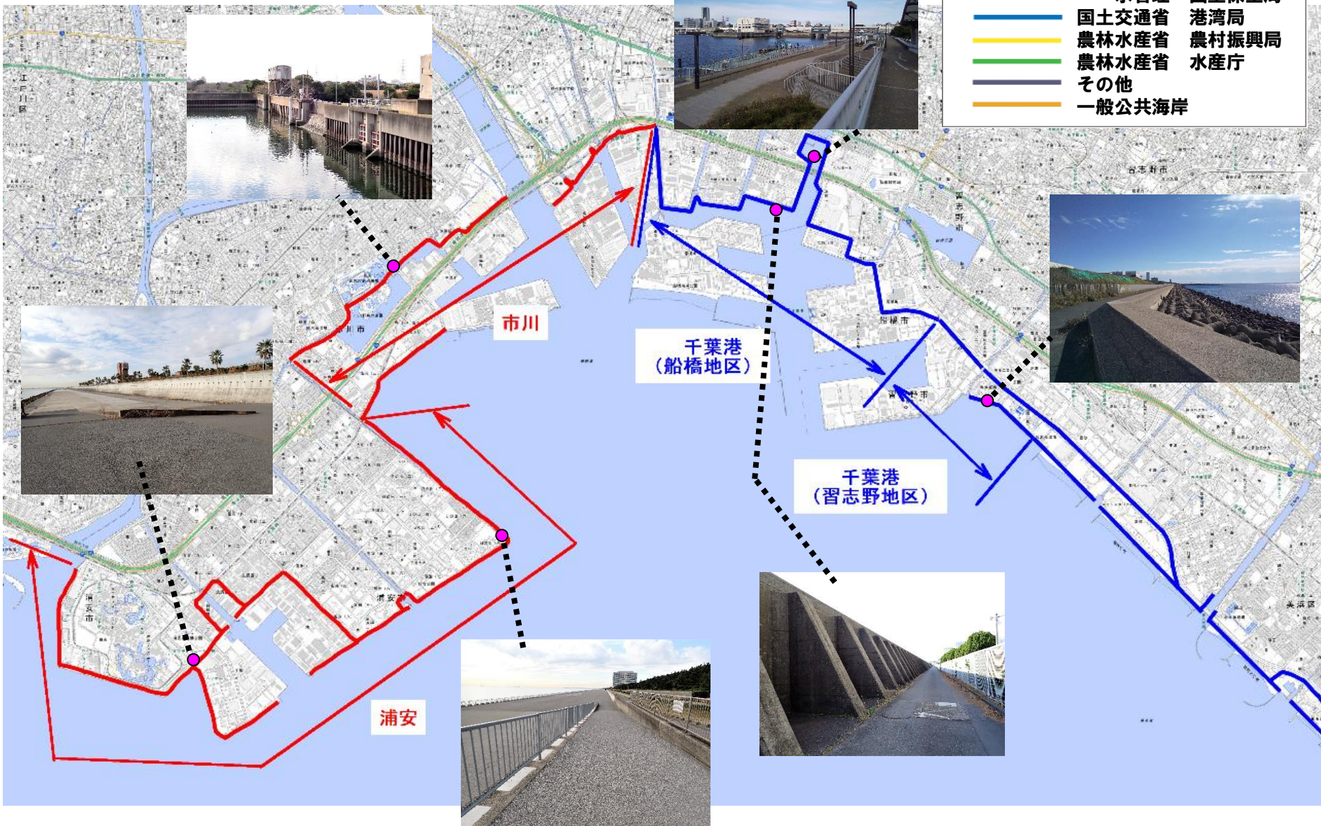
図 1-1.10 東京湾沿岸における現況の海岸保全区域図 (千葉港 (習志野地区) ~浦安)
