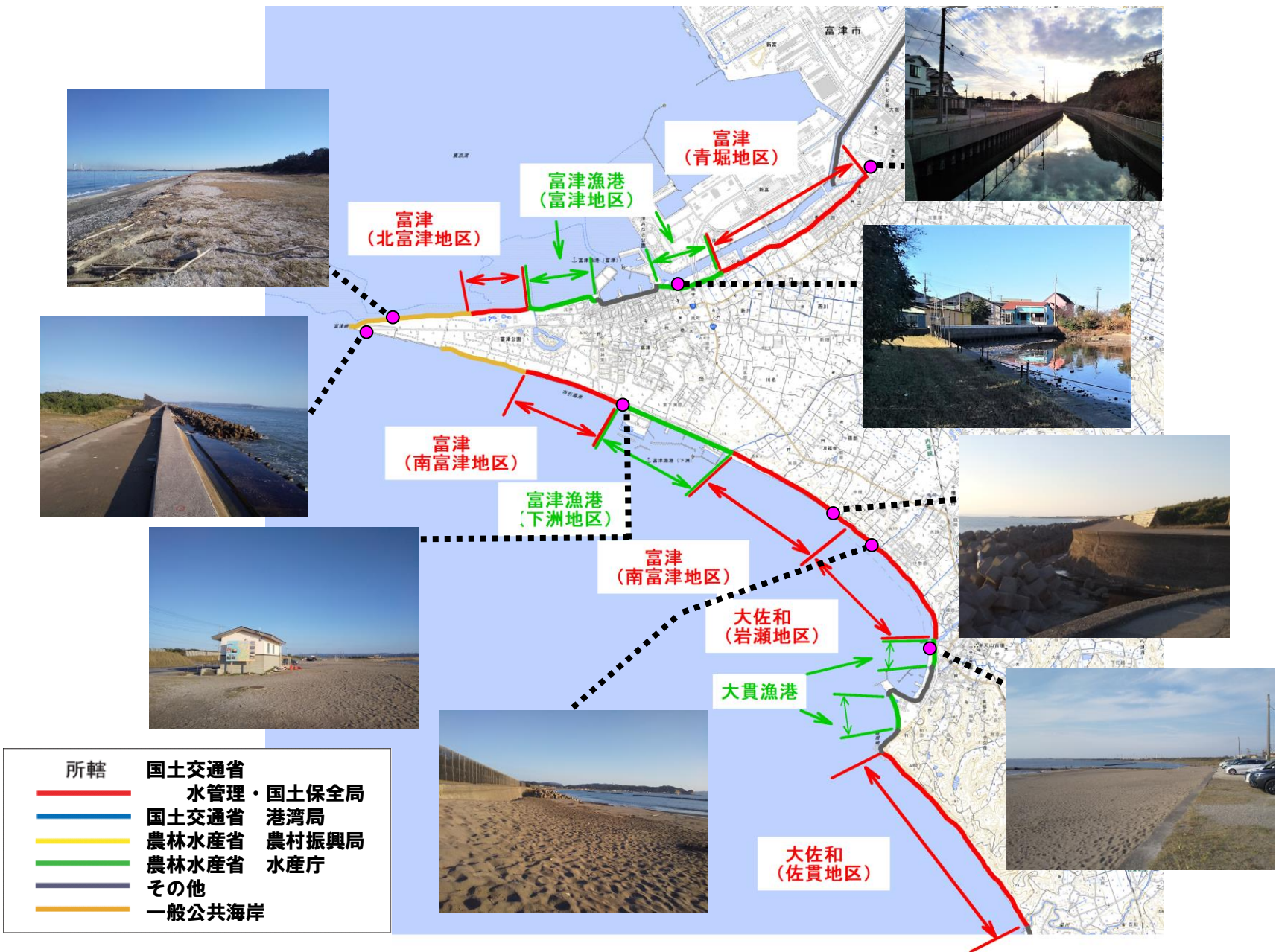
図 1-1.6 東京湾沿岸における現況の海岸保全区域図 (大佐和～富津)
