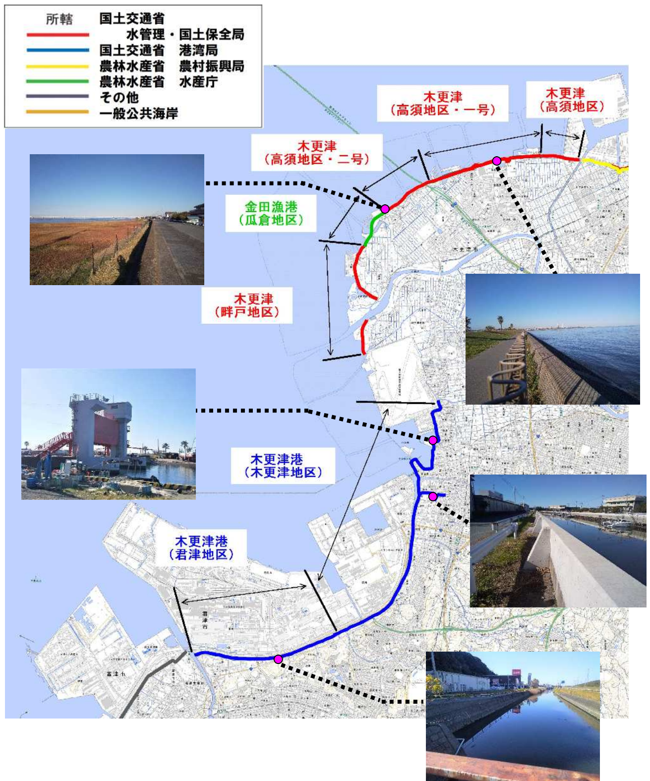
図 1 - 1.7 東京湾沿岸 [千葉県区間] における現況の海岸保全区域図 (木更津港 (君津地区) ~木更津 (高須地区)) 背景地図の出典：国土地理院地図 (淡色地図)
