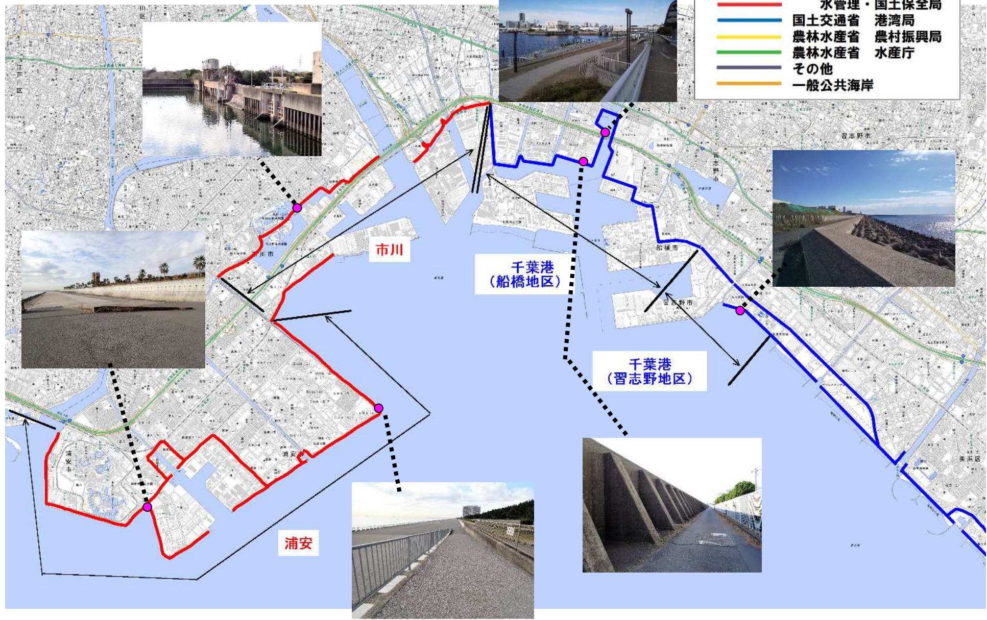
図 1-1.10 東京湾沿岸「千葉県区間」における現況の海岸保全区域図（千葉港（習志野地区）～浦安）
