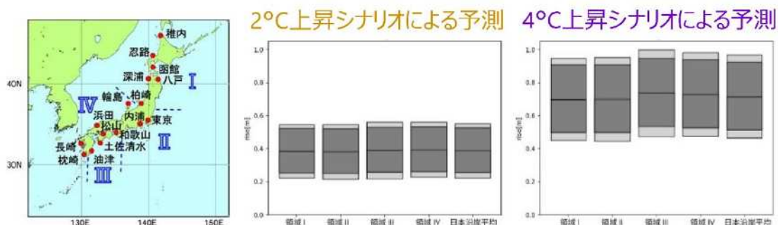
図 1－2.8 1986～2005 年を基準とした、 21 世紀末における日本沿岸平均海面水位上昇の変化予測
