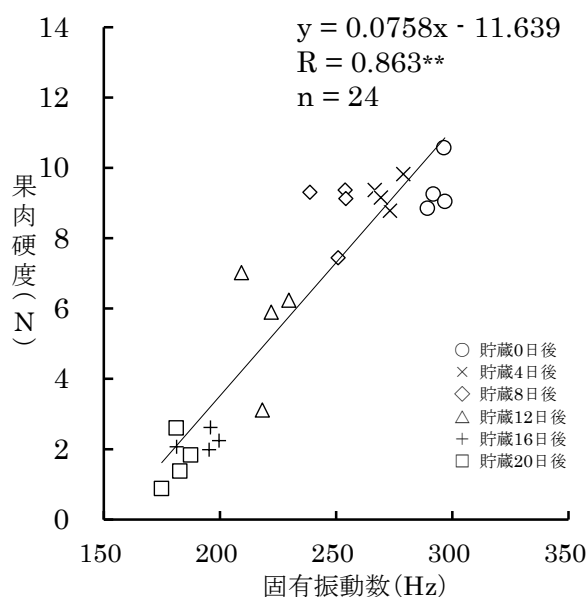
第1図 2014年収穫の「タカミ」(小型ハウス栽培)における固有振動数と果肉硬度の関係
