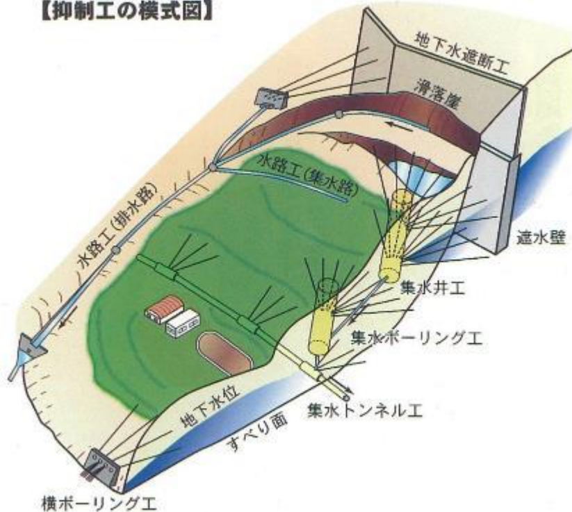
【抑制工の模式図】
