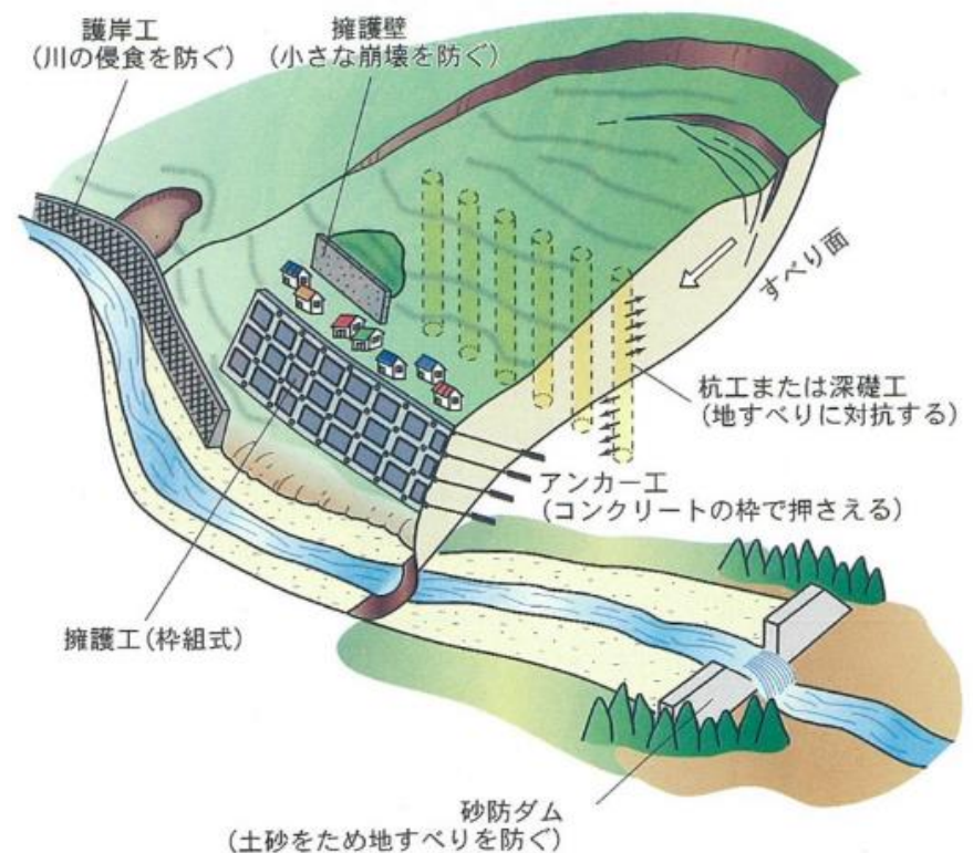
【抑止工模式図】(力学的な抑制工含)
