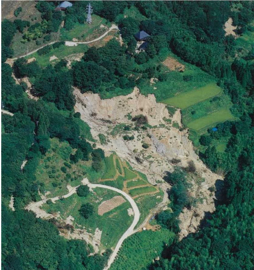
平成元年 鋸南町小保田北地区の大規模地すべり
