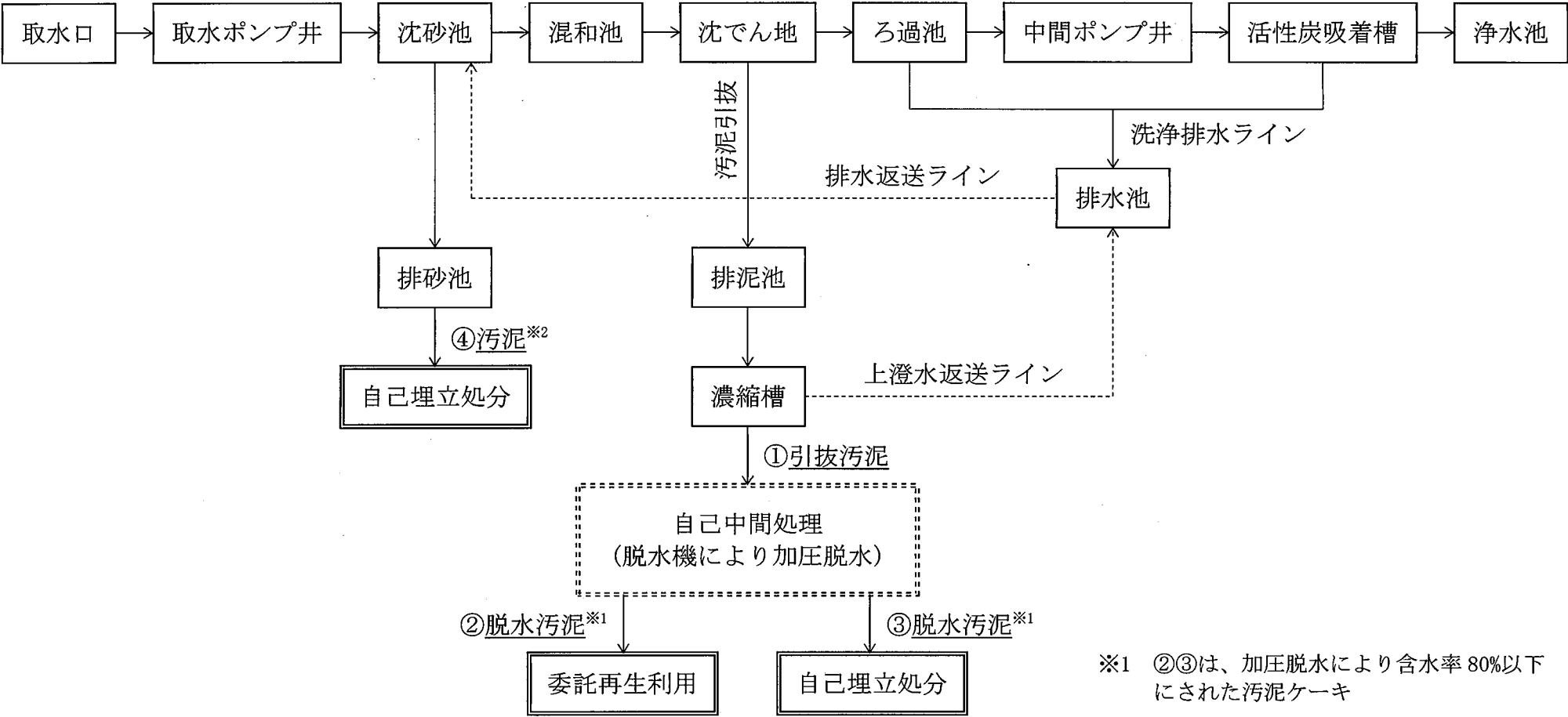
浄水処理工程図（大寺浄水場）
