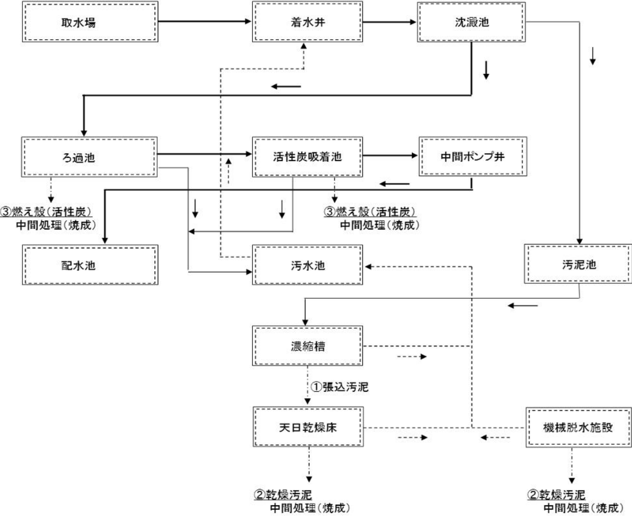
浄水処理工程図
