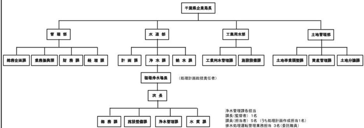
(管理体制図)
