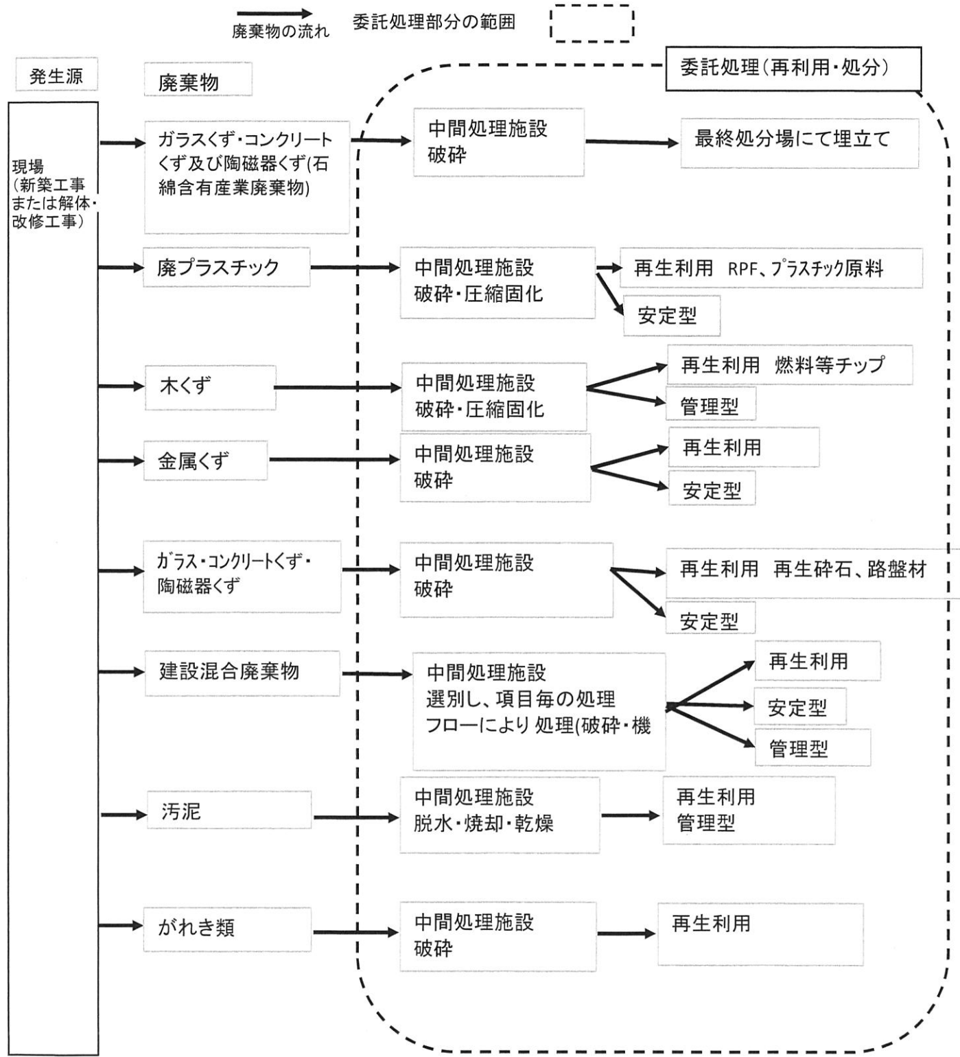
別紙1 廃棄物処理フロー図
