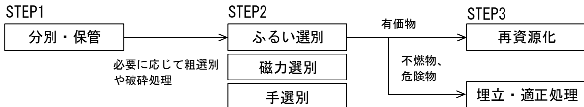
図表 II-21 金属くずの処理フロー
