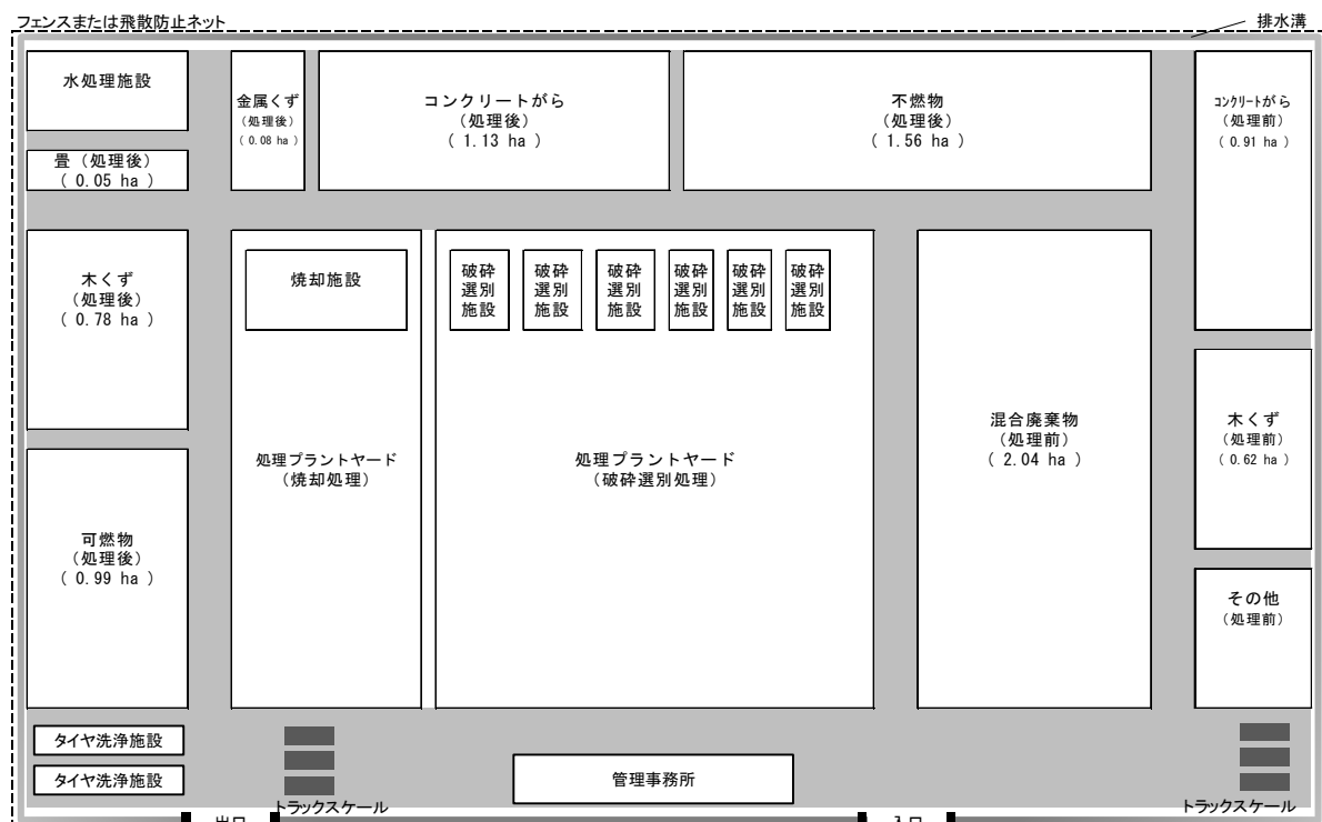
図表 III-77 二次仮置場における保管ヤード及び中間プラントヤードの配置例(県内処理)
