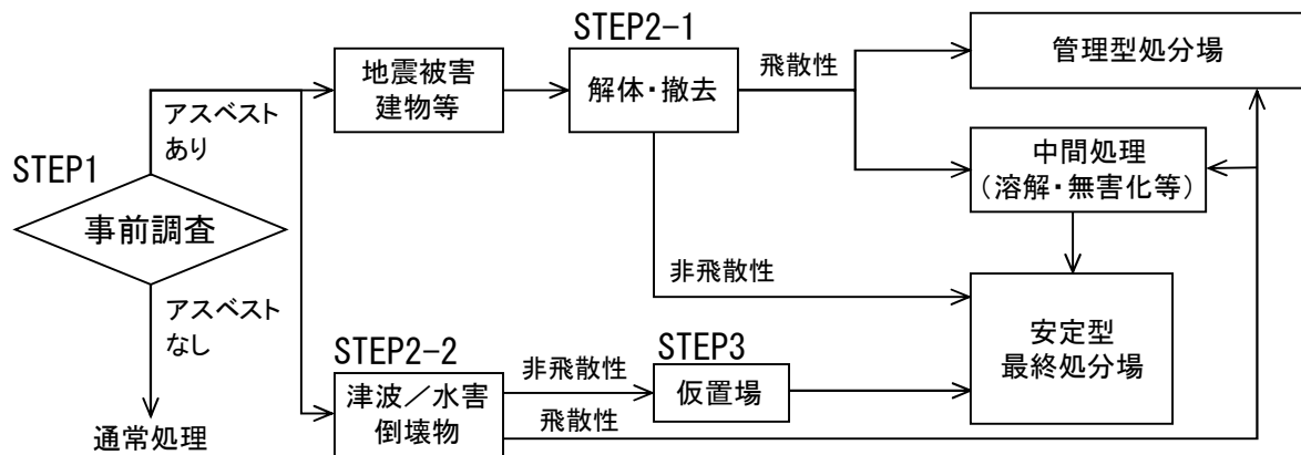
図表 Ⅱ-32 有害・危険物の処理フロー
