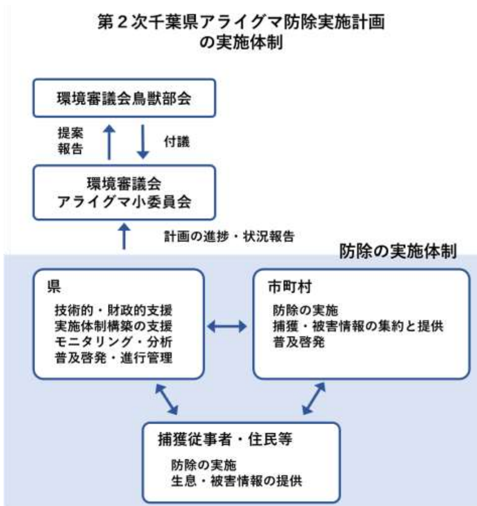
図 12. 実施体制図
