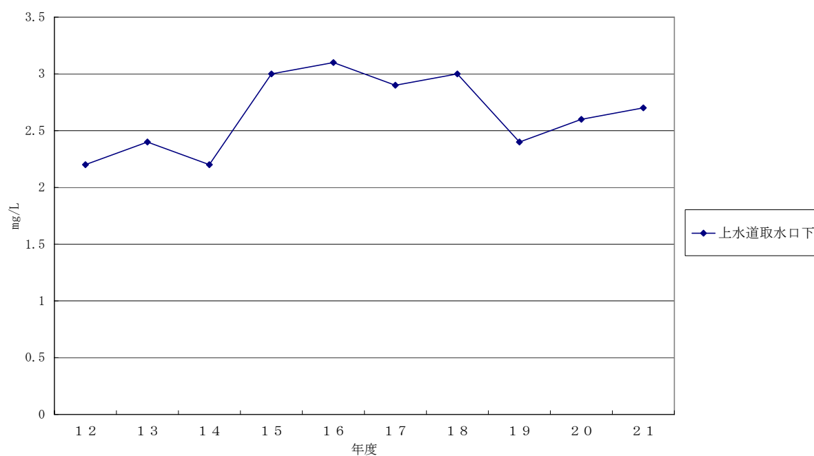
図1-18 全窒素推移
