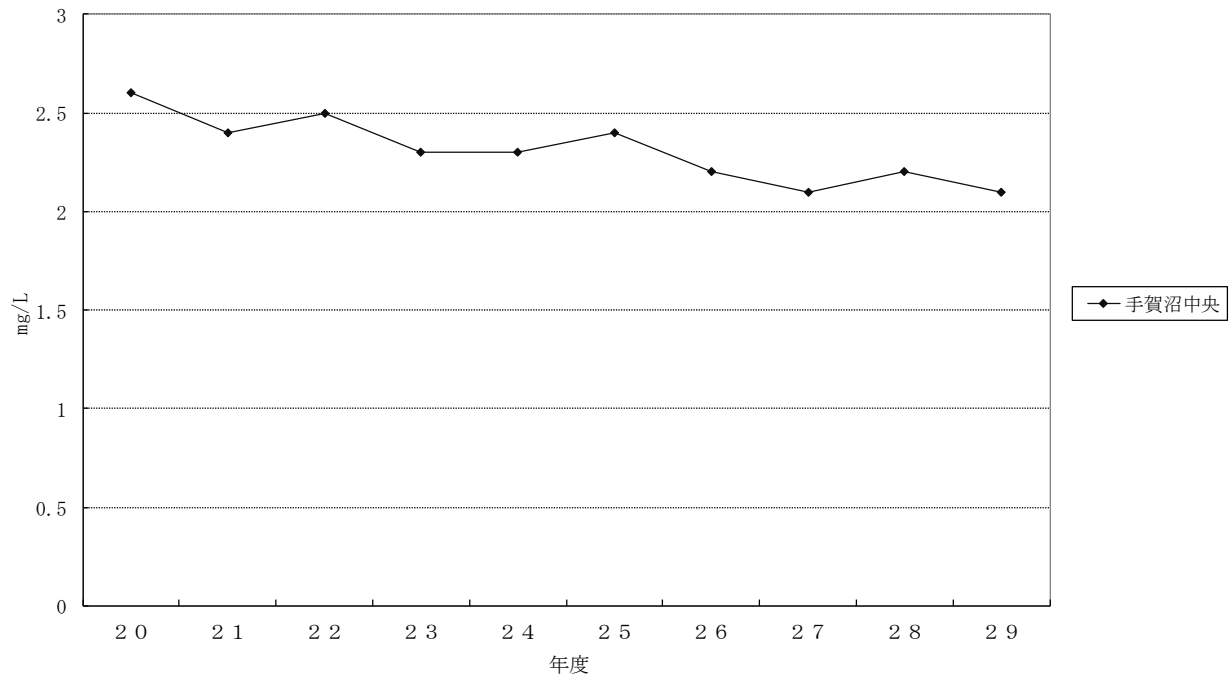
図1-22 全窒素推移
