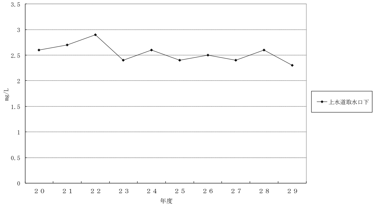
図1-18 全窒素推移
