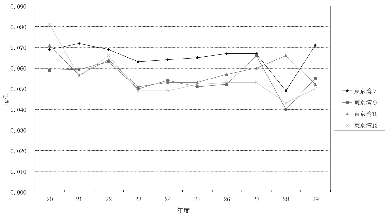
図1-27 全りん推移
