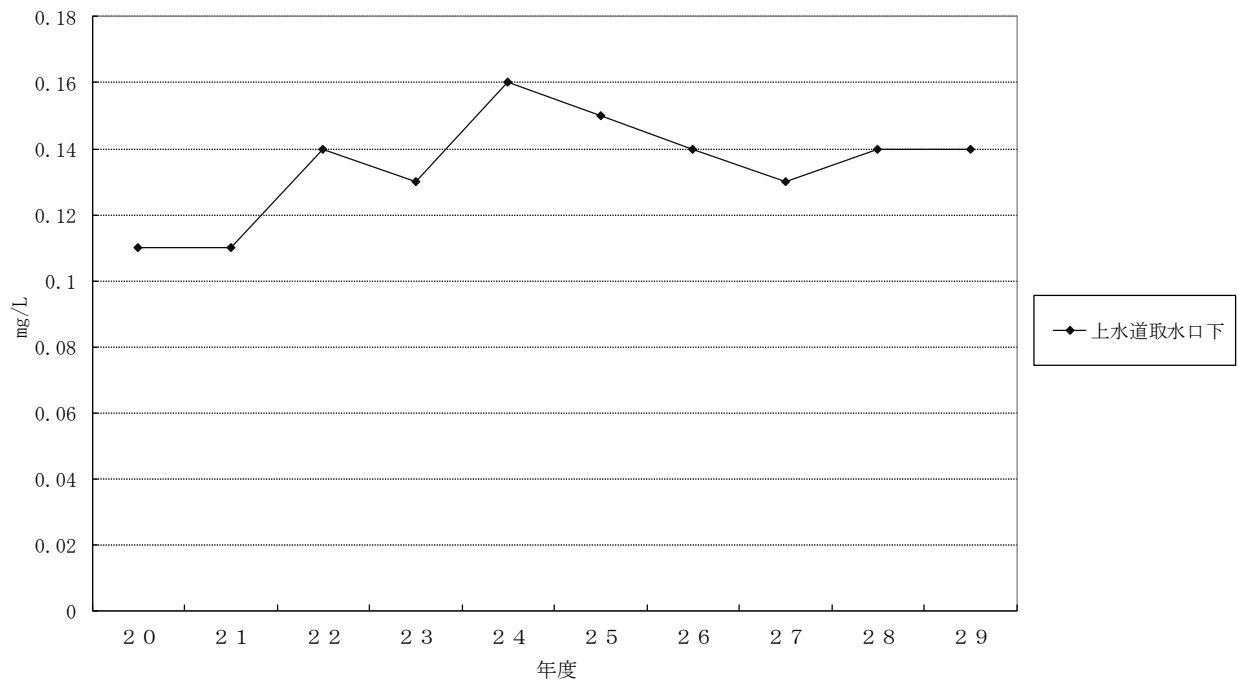
図1-19 全りん推移
