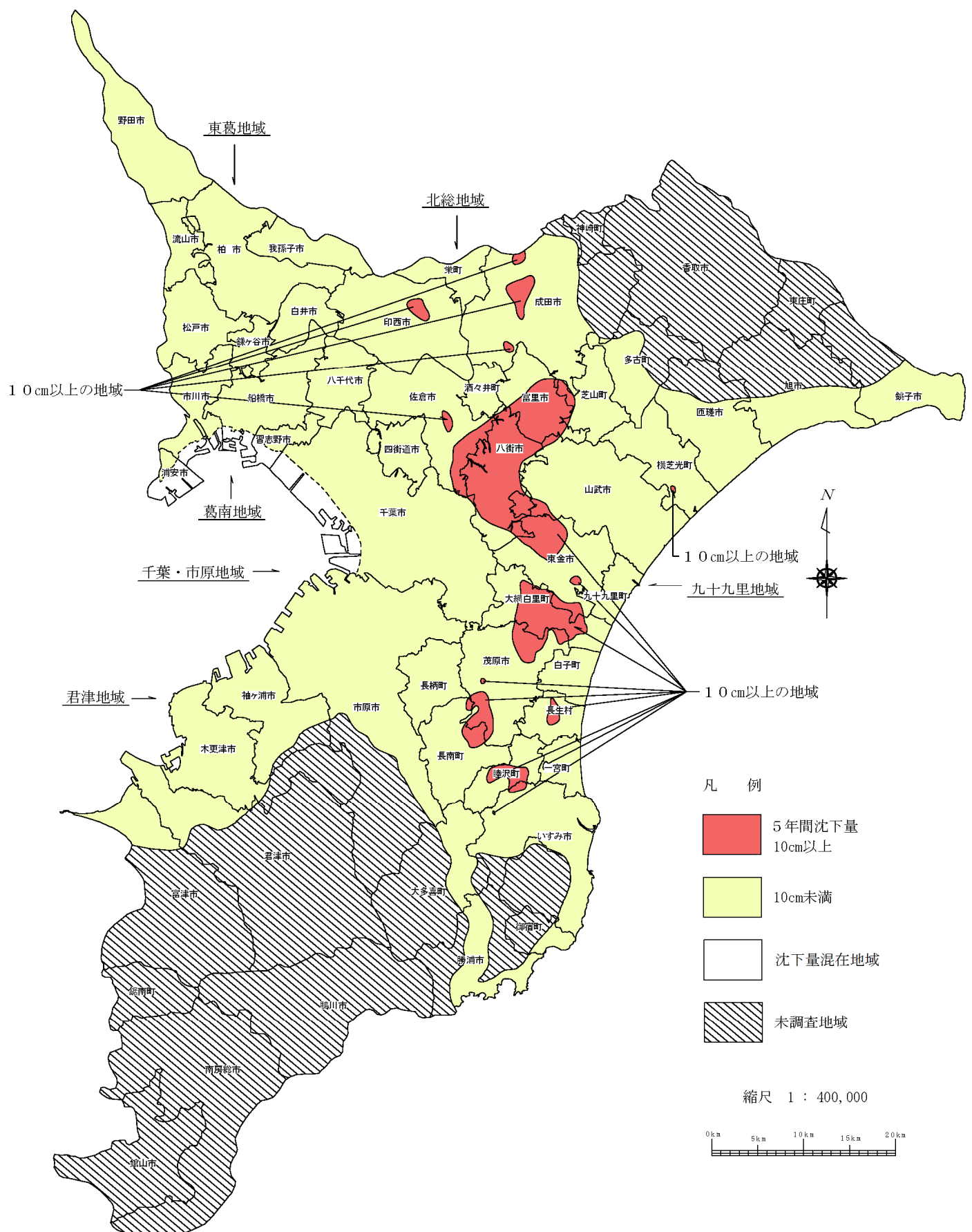
図2 千葉県水準基標変動図 (5年間変動図) (平成19年1月～平成23年11月-平成24年3月)
