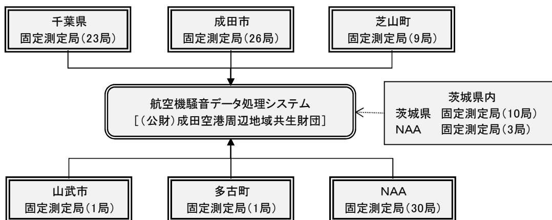
図２ 測定局と共生財団システムの構成
