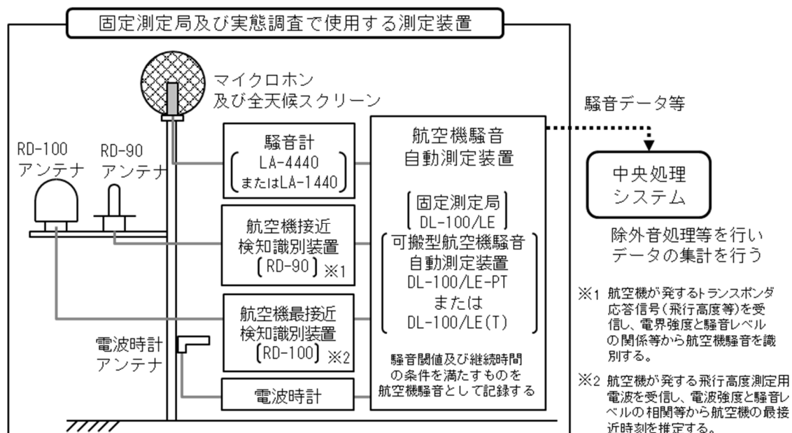
図2 基本構成図
