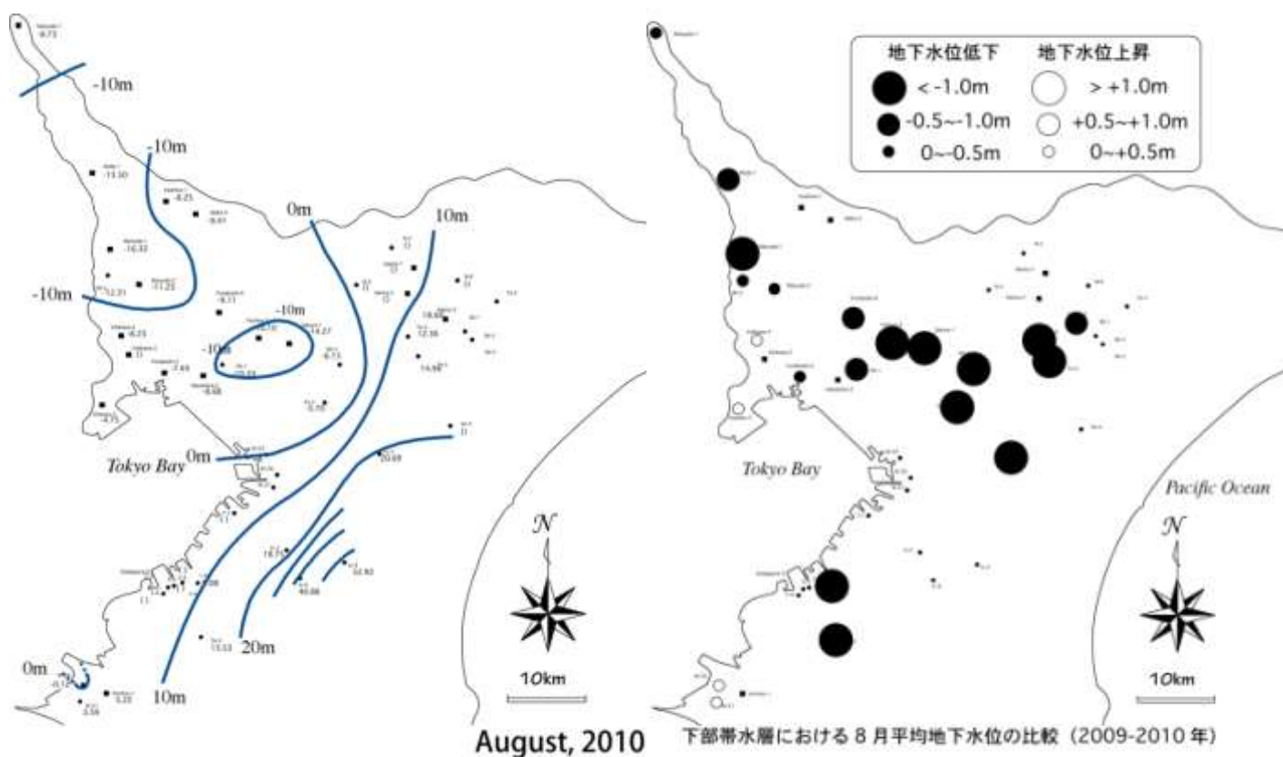
Fig. 1 下部帯水層における地下水位
