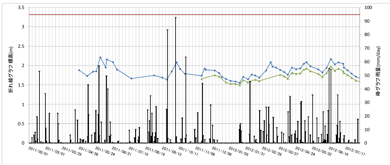
図3：埋立地（千葉県環境研究センター）における地下水位標高（T.P.） 赤：地表 青：埋立地層の地下水位 緑：沖積層の地下水位 黒：千葉市の日量降水量（mm/day）
