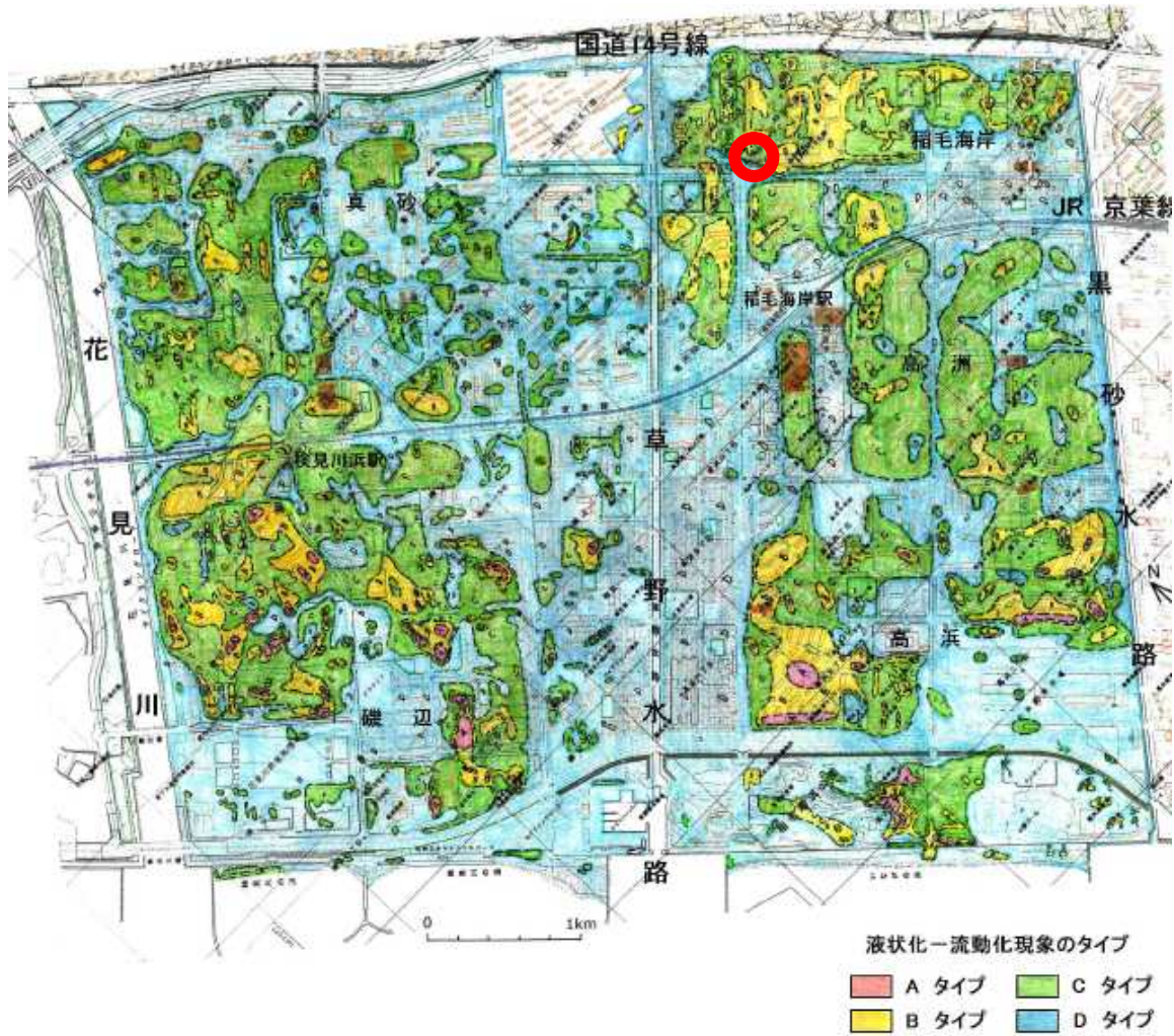
図2：調査地および液状化—流動化による変形程度（千葉県環境研究センター、赤丸）
