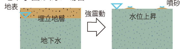
図1：地下水位の高低による液状化の起こりやすさ
