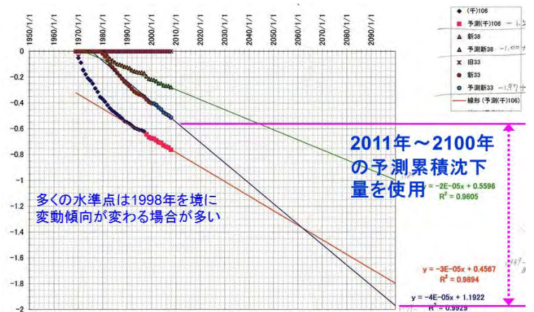
図1 白子町の水準点（千）106・新38・新33の変動状況と2100年の予測累積沈下。縦軸は変動量（m）。
