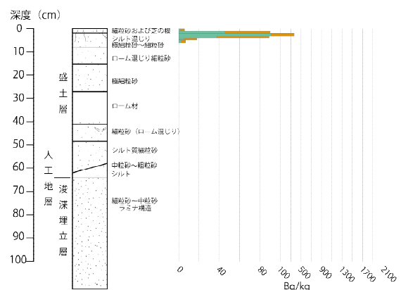
図2：2013年10月千葉市美浜区の放射性Cs測定の結果
