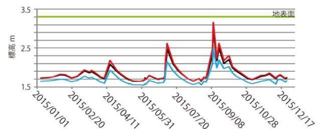
図 1：2015 年の地下水位の変化
