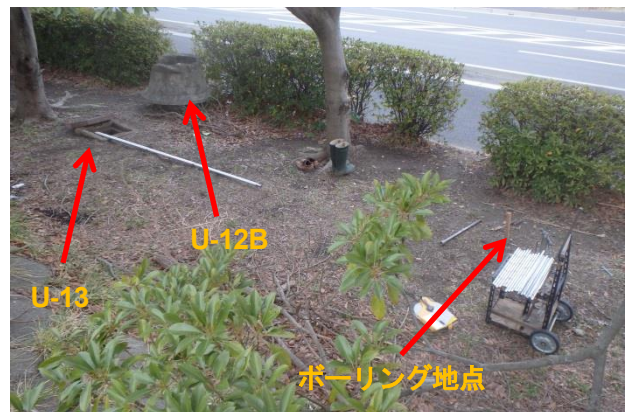
図 2 ボーリング地点付近の水準点の状況。U-13 は通常の水準点で、基礎の深さは約 1m。U-12B は基礎の深さが 10m ある水準点のため丸い杵が抜け上がっている。
