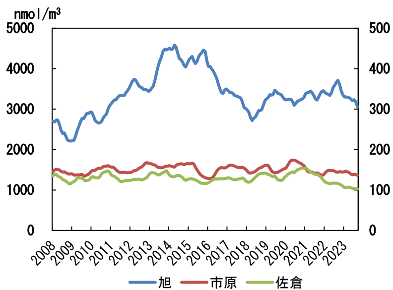
図7 PS法によるNH 3 濃度推移（旭は左軸、市原及び佐倉は右軸）
