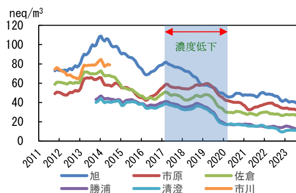
図 5 \text{F}_0 粒子中 \text{NH}_4^+ 当量濃度推移
