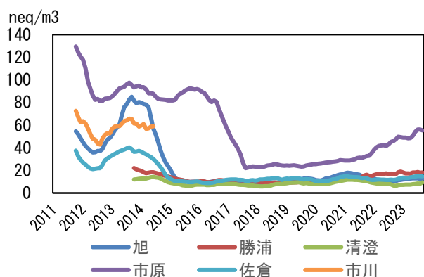
図 6 \text{F}_0 粒子中 \text{nss-Ca}^{2+} 当量濃度推移
