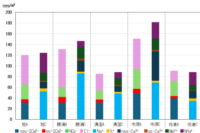
図 3 各地点の粒子状物質中のイオン成分の当量濃度（nss-：非海塩性イオン、ss-：海塩性イオン）
