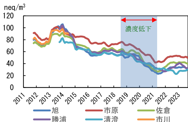
図 4 \text{F}_0 粒子中 \text{nss-SO}_4^{2-} 当量濃度推移
