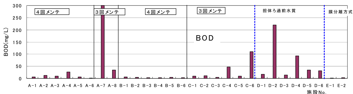
図1 施設別処理水BOD
