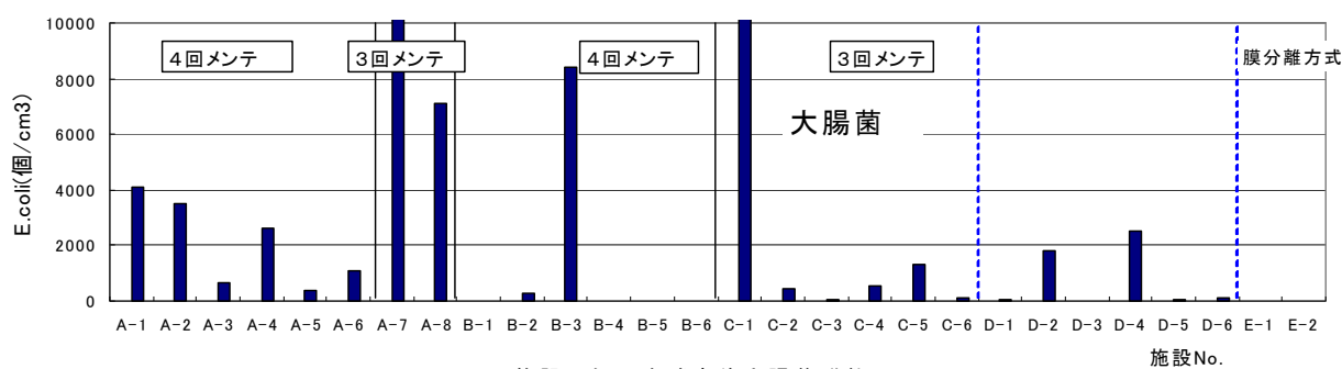
図3 施設別処理水消毒後大腸菌群数
