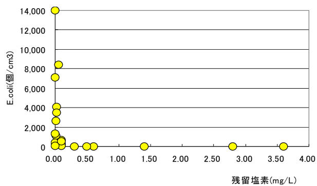
図4 残留塩素と大腸菌群数の関係1
