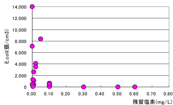
図5 残留塩素と大腸菌群数の関係2
