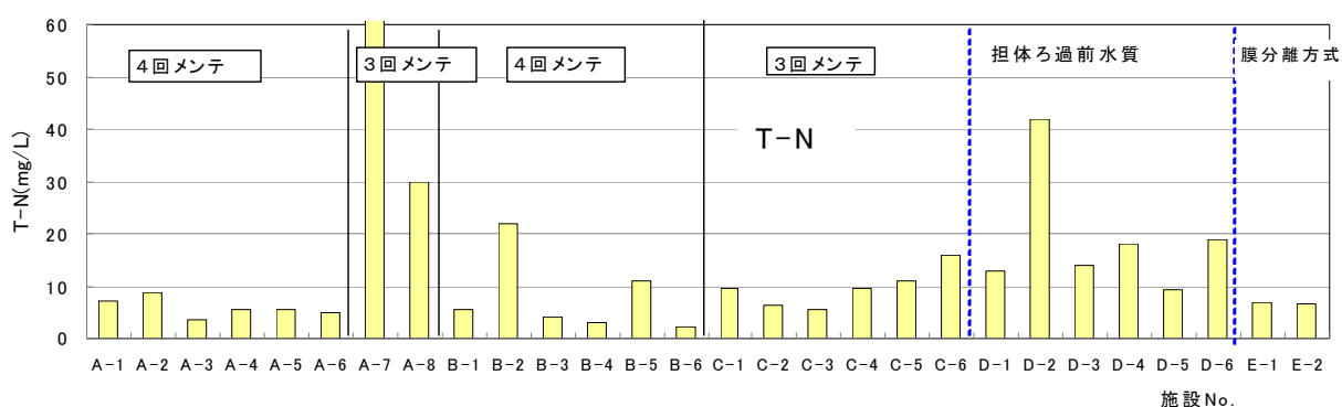
図2 施設別処理水T-N
