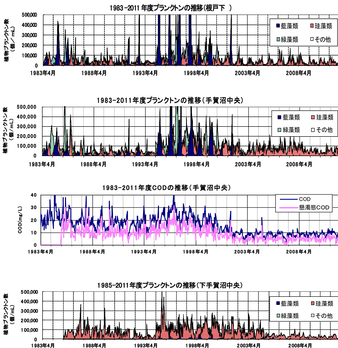
図2 各測定地点の網別プランクトン数と手賀沼中央水質 (COD) の変化
