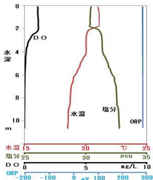
図2 6/13 船橋港の水質鉛直プロファイル
