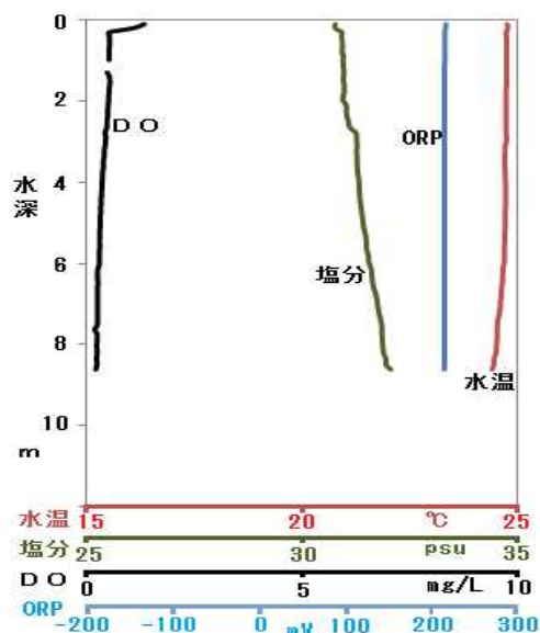
図3 9/24 船橋港の水質鉛直プロファイル
